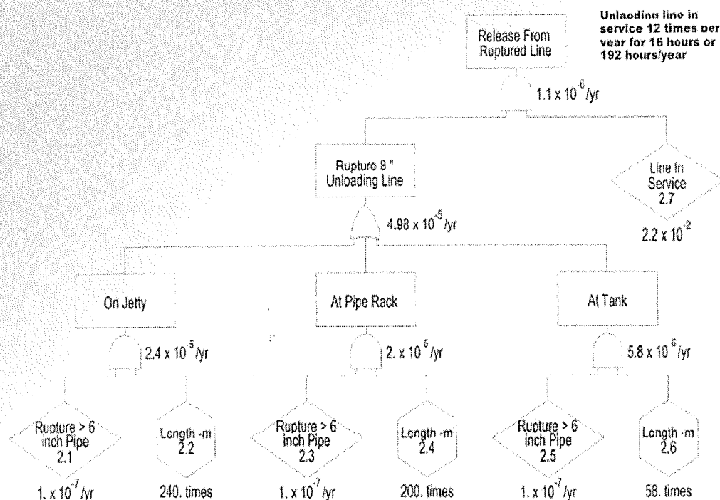
Slika 29 Primjer analize mogućih scenarija havarije metodom "Fault Tree"
