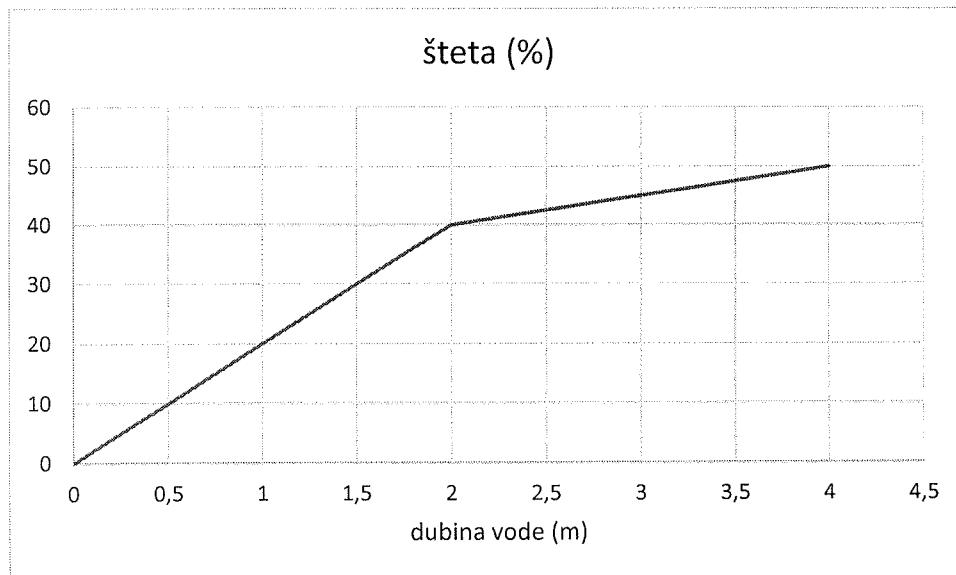
Slika 30 Krivulja štete od poplave „stock in trade industry“
