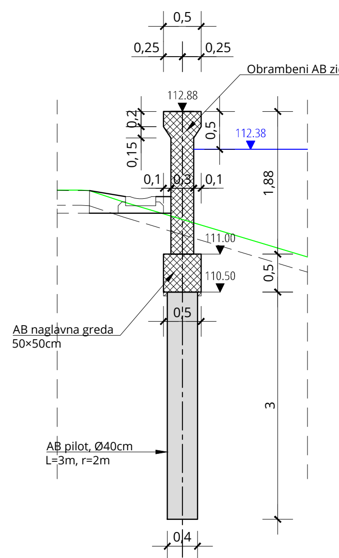
PRESJEK B-B MJ 1:50
