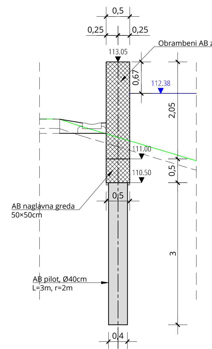
PRESJEK C-C MJ 1:50
