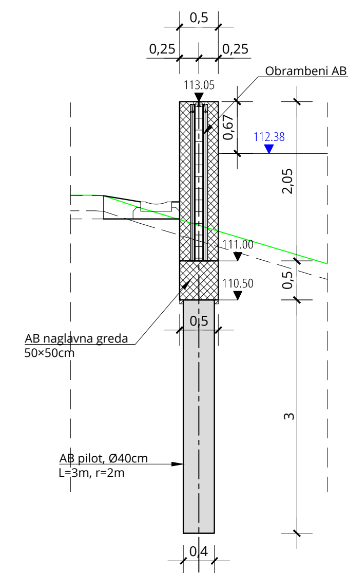
PRESJEK D-D MJ 1:50
