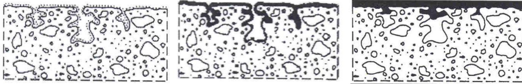
Slika 7-03.3.2.-1 Shematski prikaz tipične hidrofobne impregnacije (lijevo), impregnacije (sredina) i premaza (desno)
