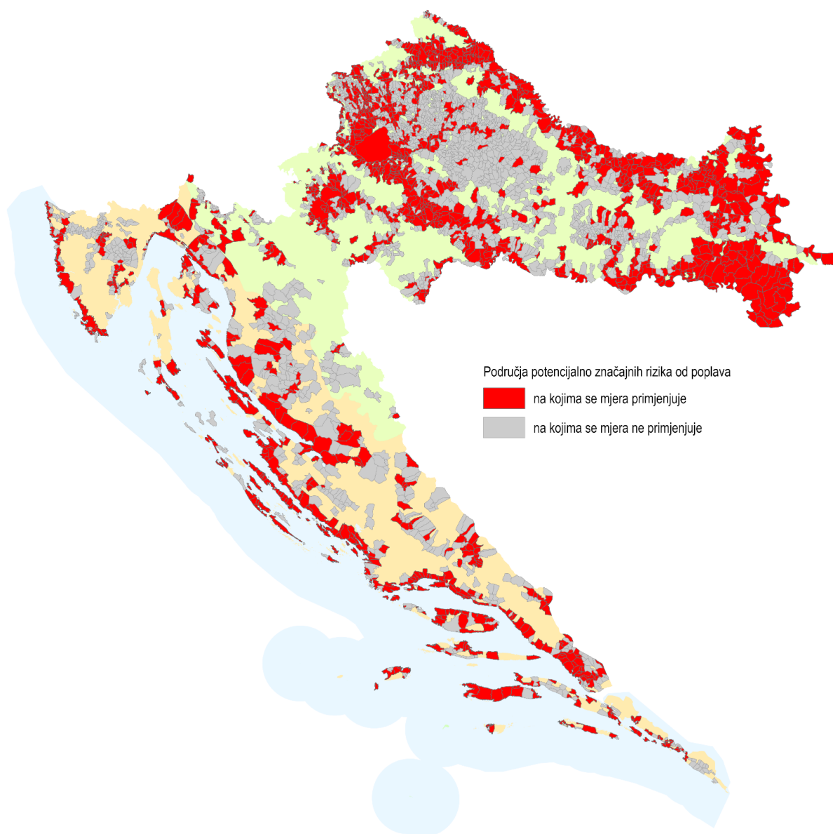
Sl. 1 Područja potencijalno značajnih rizika od poplava na koje se odnosi mjera 3.URP.23.B
