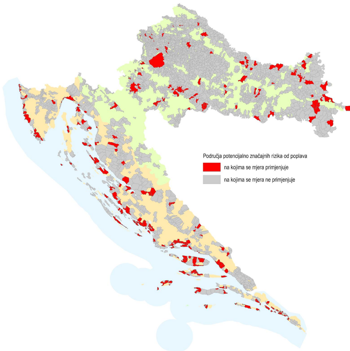
Sl. 4 Područja potencijalno značajnih rizika od poplava na koje se odnosi mjera 3.URP.SM6
