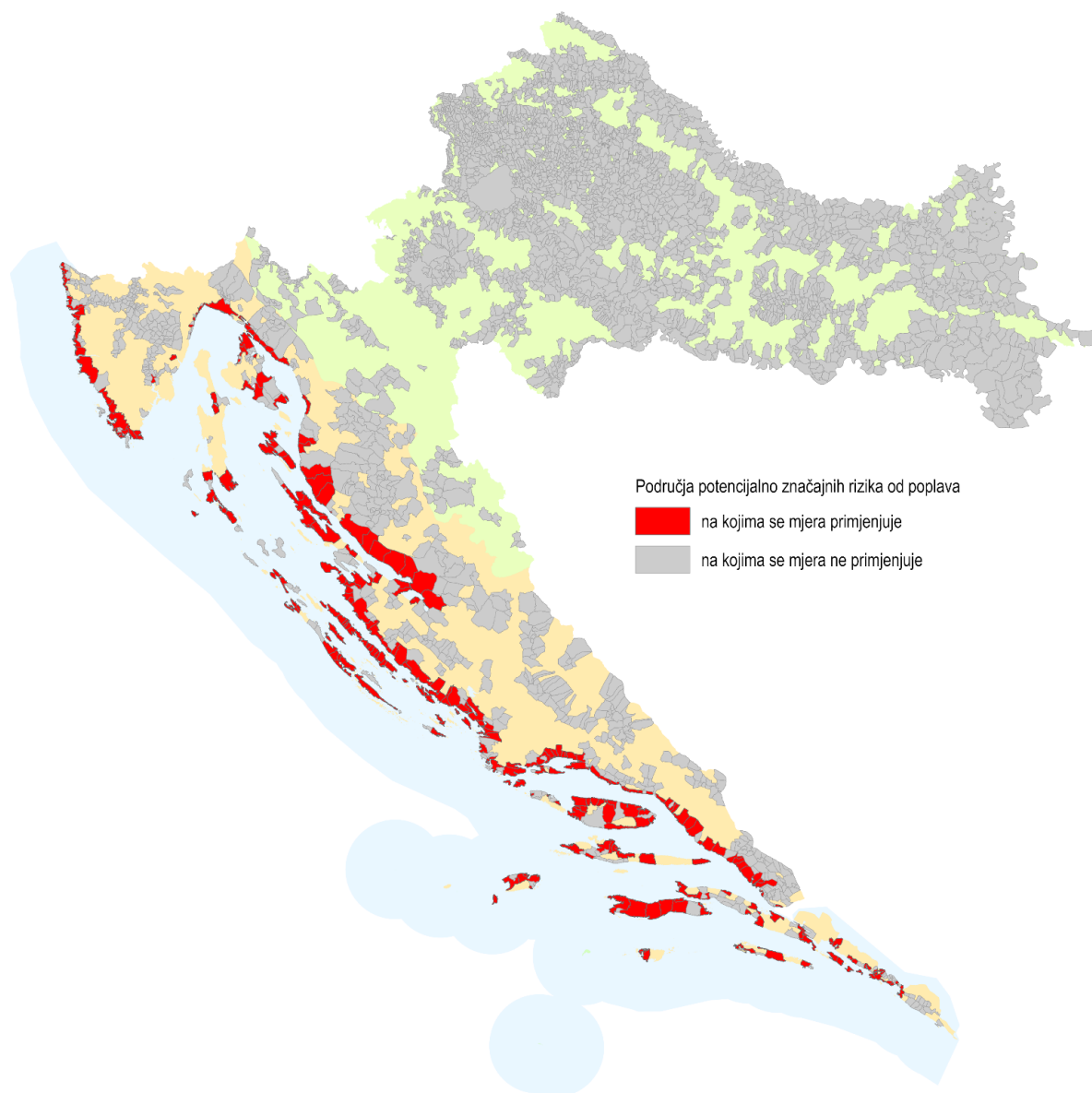
Sl. 2 Područja potencijalno značajnih rizika od poplava na koje se odnosi mjera 3.URP.25
