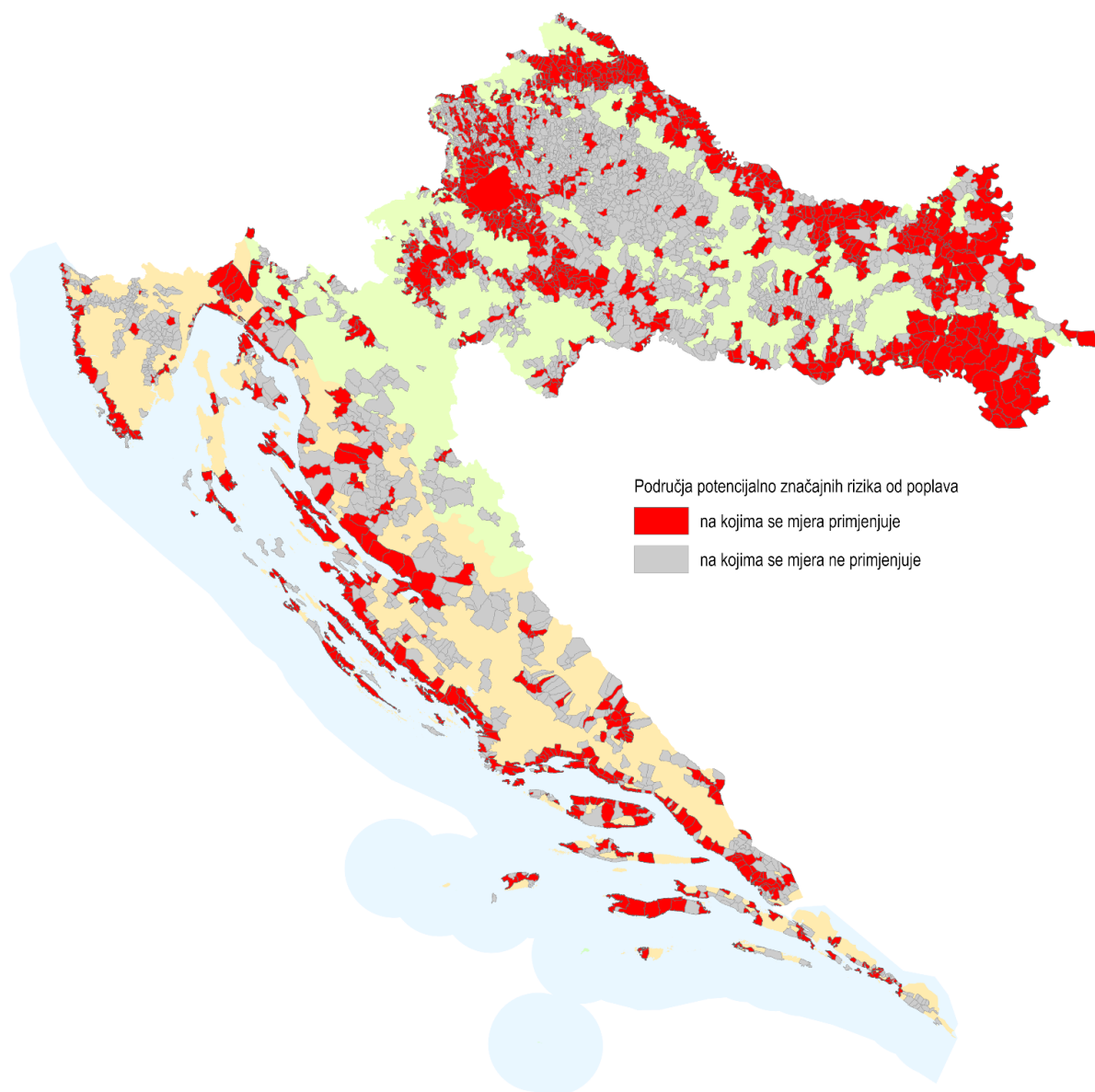
SI. 3 Područja potencijalno značajnih rizika od poplava na koje se odnose mjere 3.URP.42.A i 3.URP.43.A
