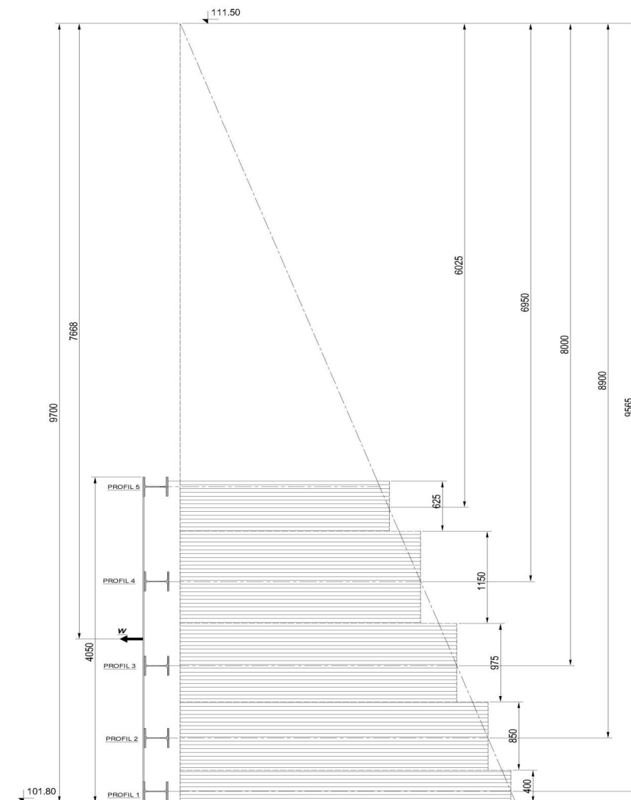
Slika 1. Raspodjela hidrostatske sile po raspoređenim profilima
