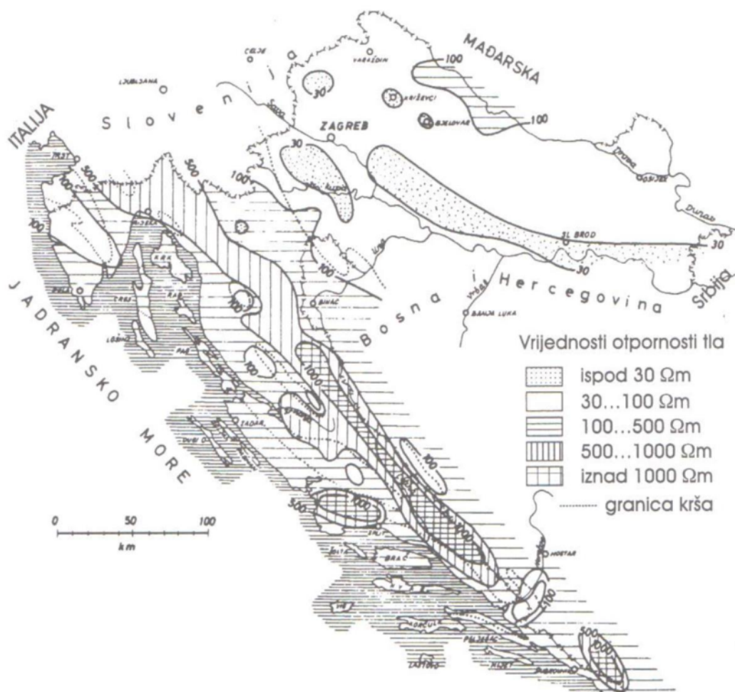
Slika 7.1: Orijentacijska karta otpornosti tla na dubini od 1 m za područje Hrvatske (izvor: Uzemljivači i sustavi uzemljenja, Majdandžić Franjo, Zagreb: Graphis, 2004.)
