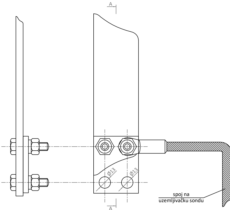
PRESJEK A-A
