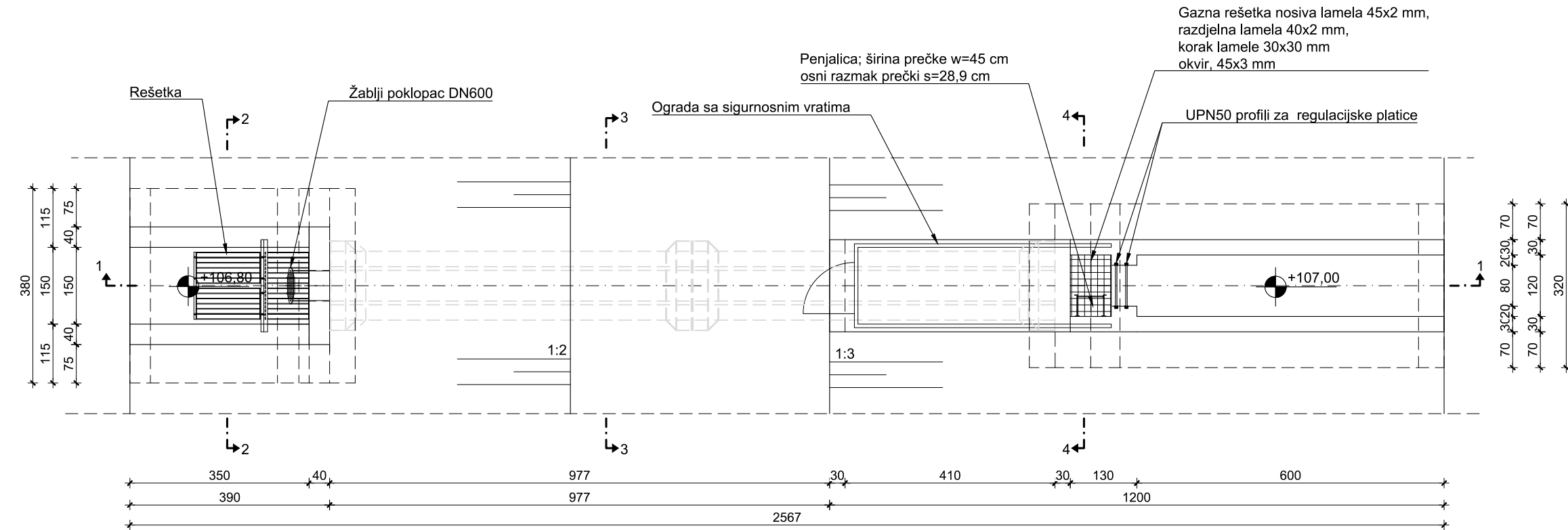
TLOCRT A-A M 1:100
