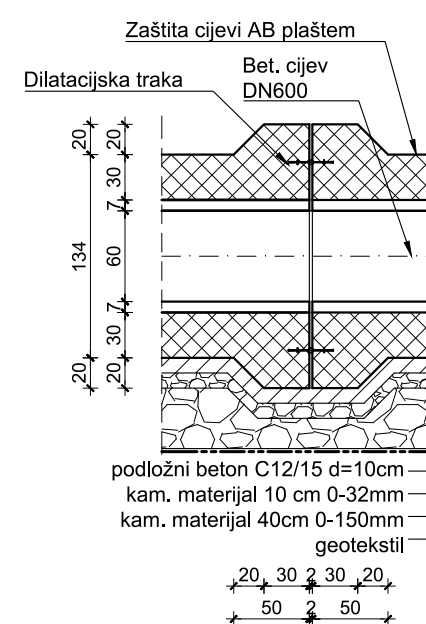
DETALJ DILATACIJE CJEVOVODA M 1:50
