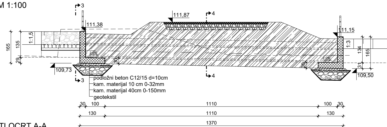
TLOCRT A-A M 1:100
