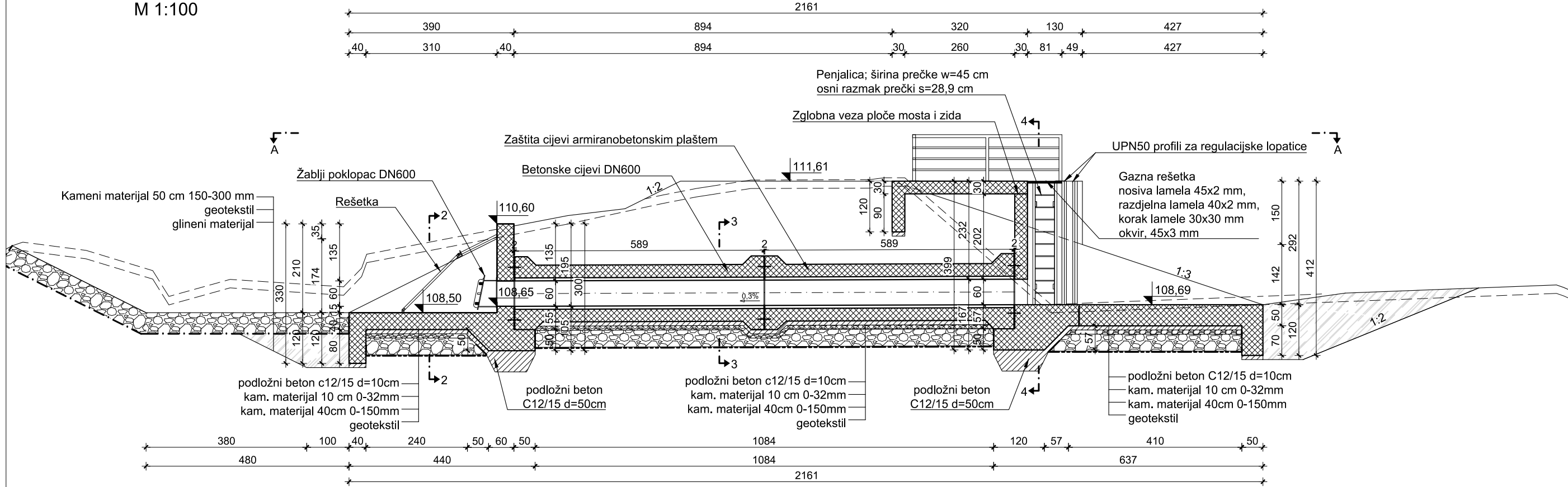
UZDUŽNI PRESJEK 1-1 M 1:100
