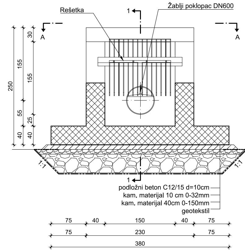
Gazna rešetka nosiva lamela 45x2 mm, razdjelna lamela 40x2 mm, korak lamele 30x30 mm okvir 45x3 mm Penjalica; širina prečke w=45 cm osni razmak prečki s=28,9 cm L profil 50 x 50 x 4 Bet. cijev DN 600 Podložni beton C12/15 d=50cm
