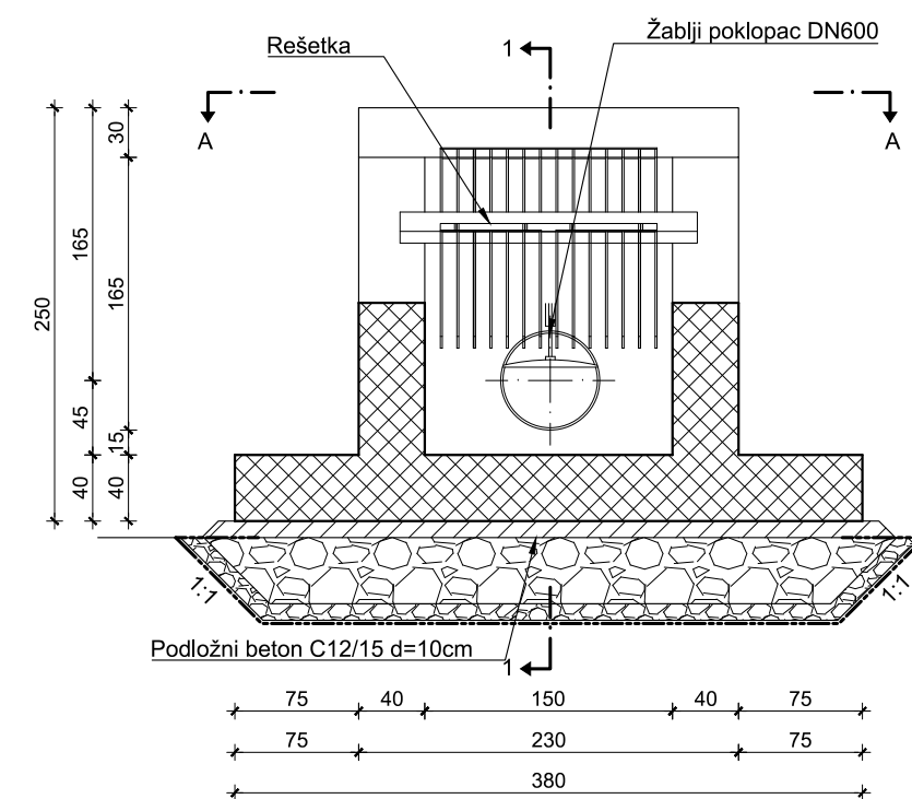
POPREČNI PRESJEK 2-2 M 1:50
