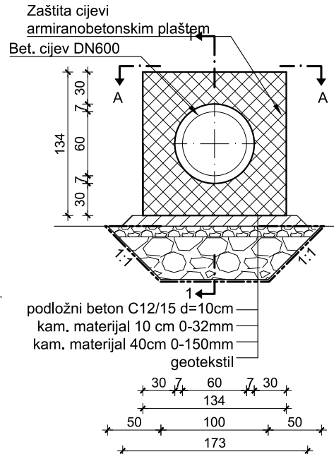
POPREČNI PRESJEK 3-3 M 1:50
