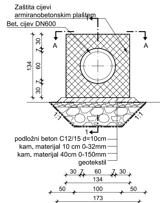
POPREČNI PRESJEK 3-3 M 1:50
