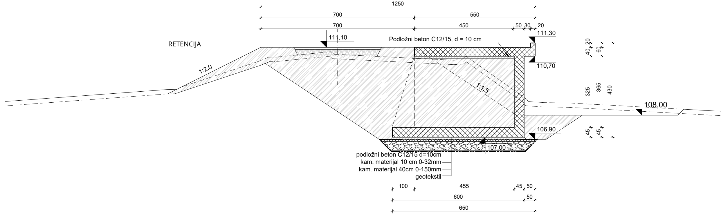
PRESJEK 1-1 M 1:100
