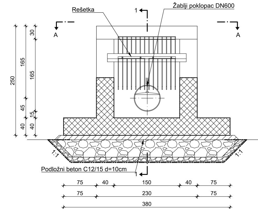
POPREČNI PRESJEK 2-2 M 1:50
