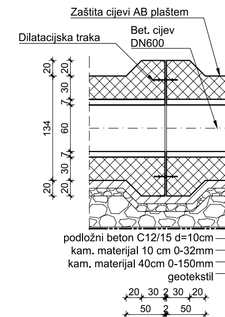
DETALJ DILATACIJE CJEVOVODA M 1:50
