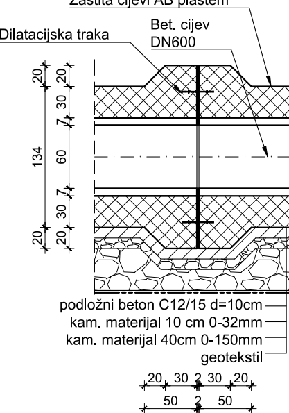
DETALJ DILATACIJE CJEVOVODA M 1:50
