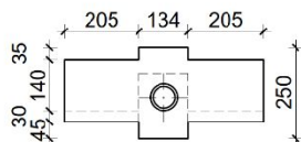
POPREČNI PRESJEK C-C
