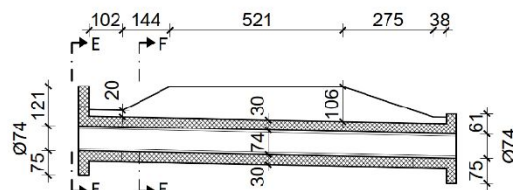
PRESJEK D-D
