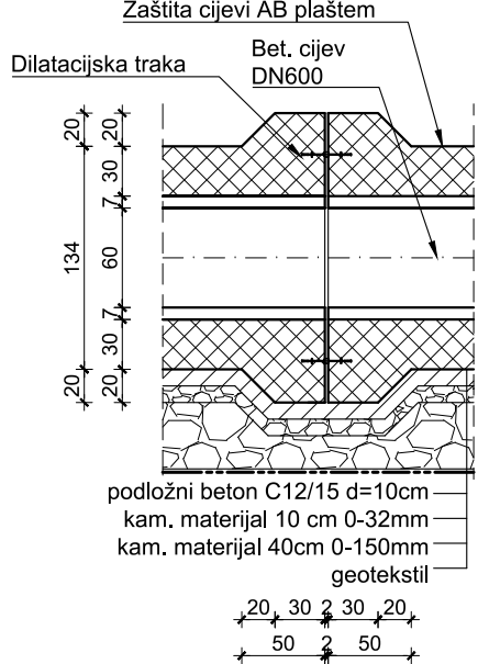
DETALJ DILATACIJE CJEVOVODA M 1:50
