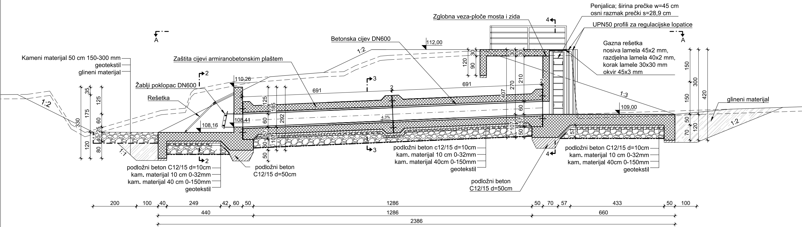
POPREČNI PRESJEK 4-4 M 1:50
