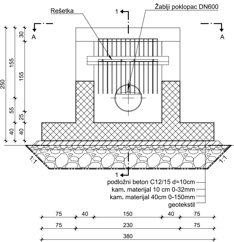
POPREČNI PRESJEK 2-2 M 1:50
