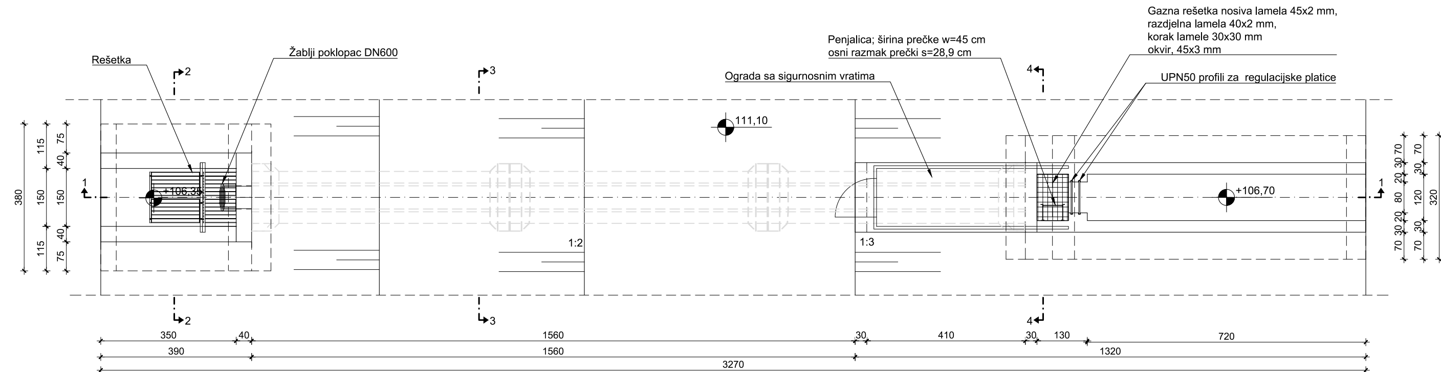
TLOCRT A-A M 1:100
