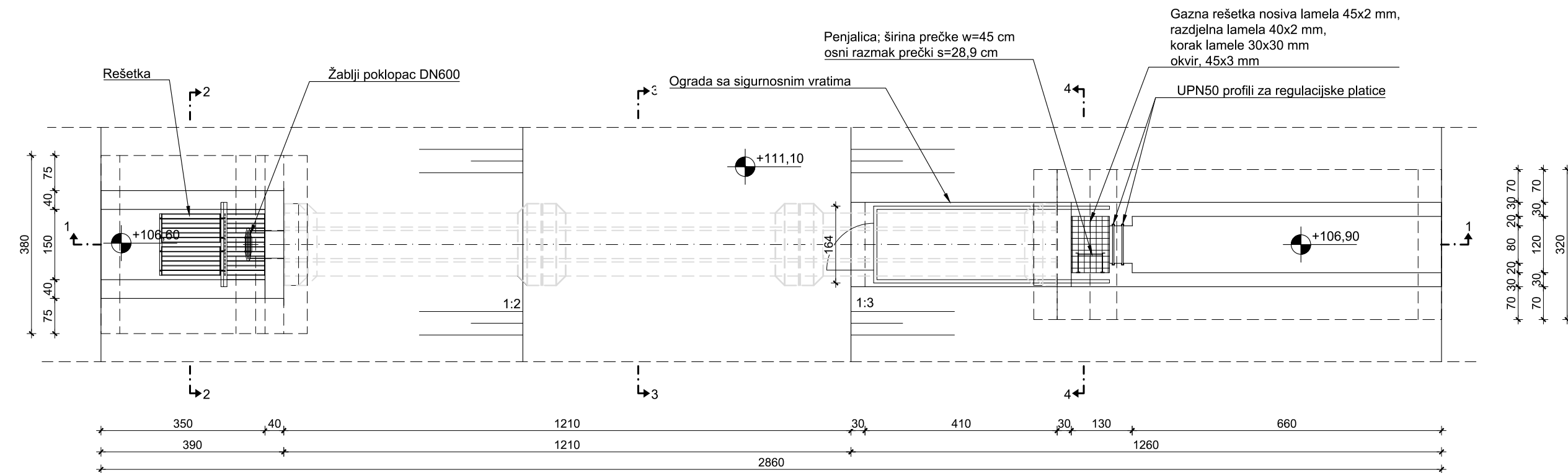
TLOCRT A-A M 1:100
