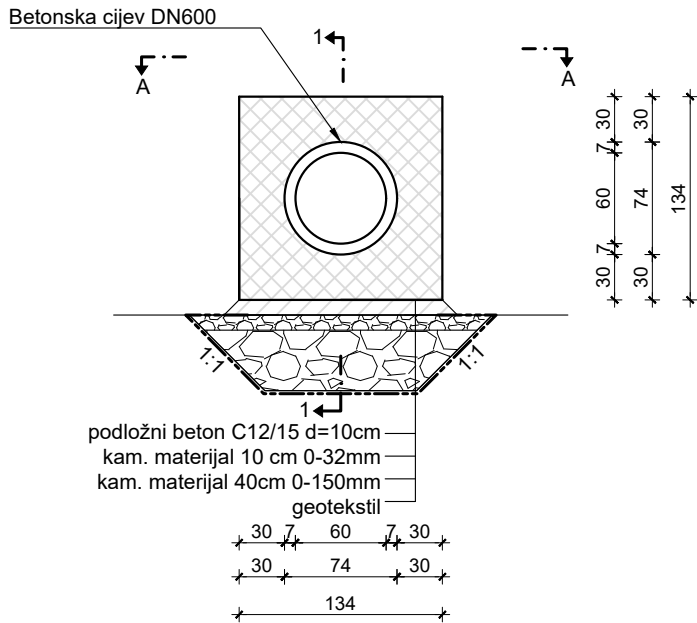
POPREČNI PRESJEK 2-2 M 1:50
