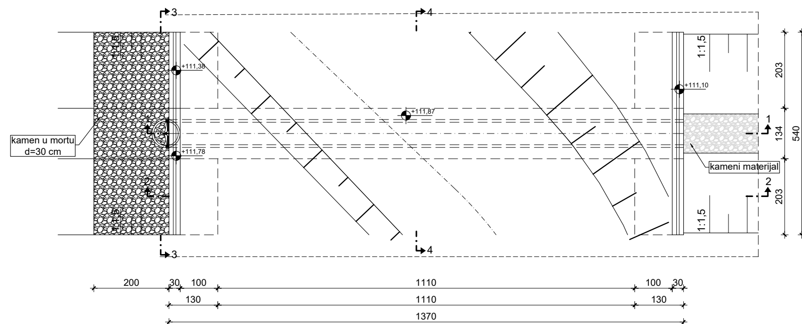
TLOCRT A-A M 1:100
