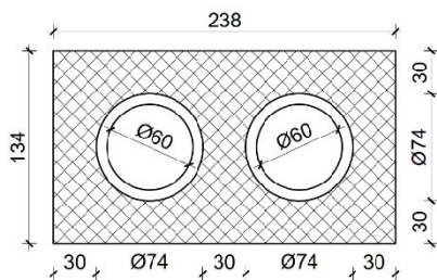
POPREČNI PRESJEK F-F
