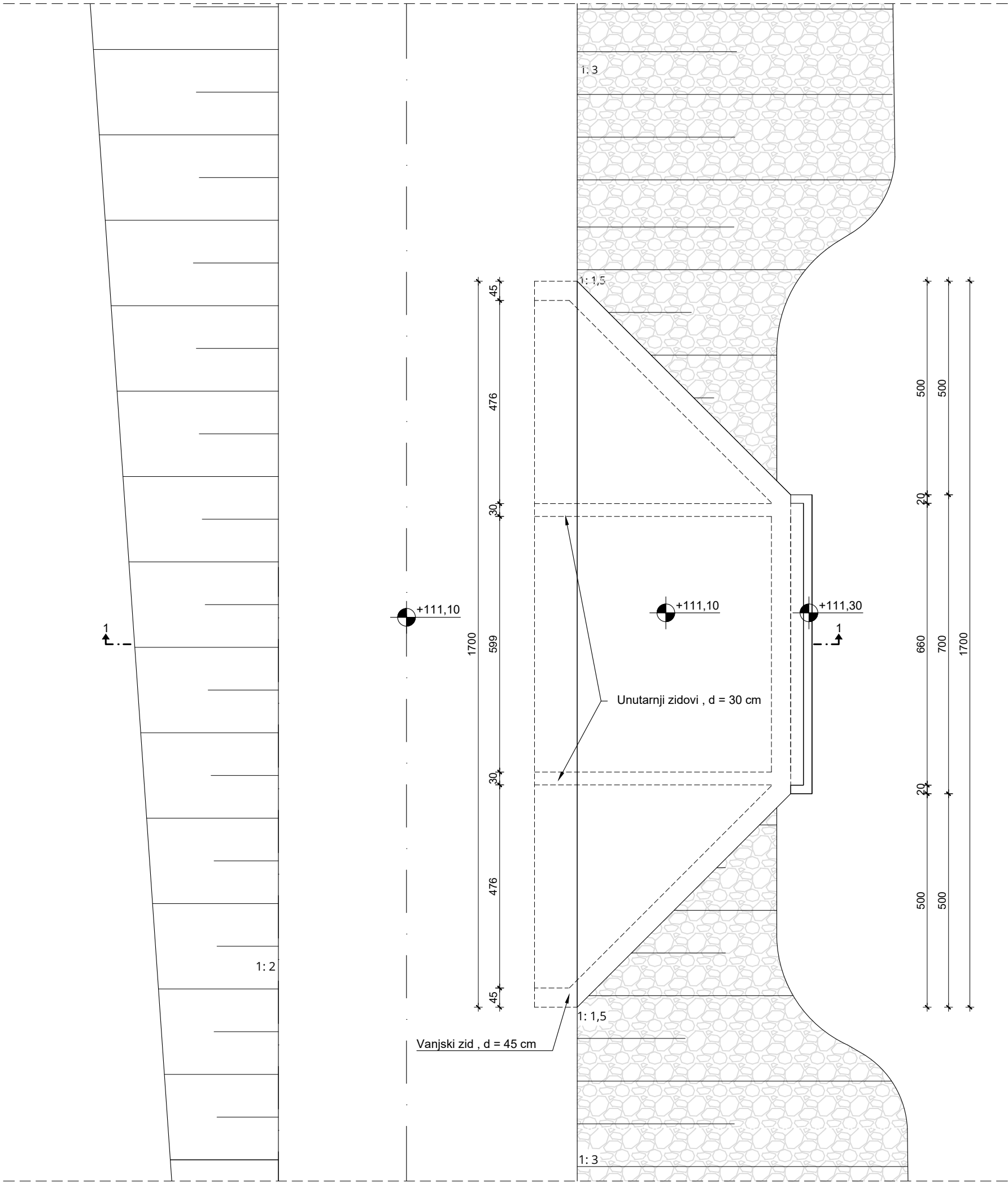
TLOCRT A-A M 1:100
