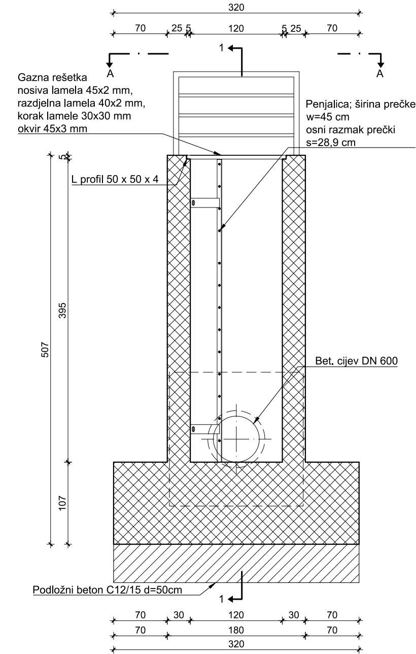
POPREČNI PRESJEK 4-4 M 1:50
