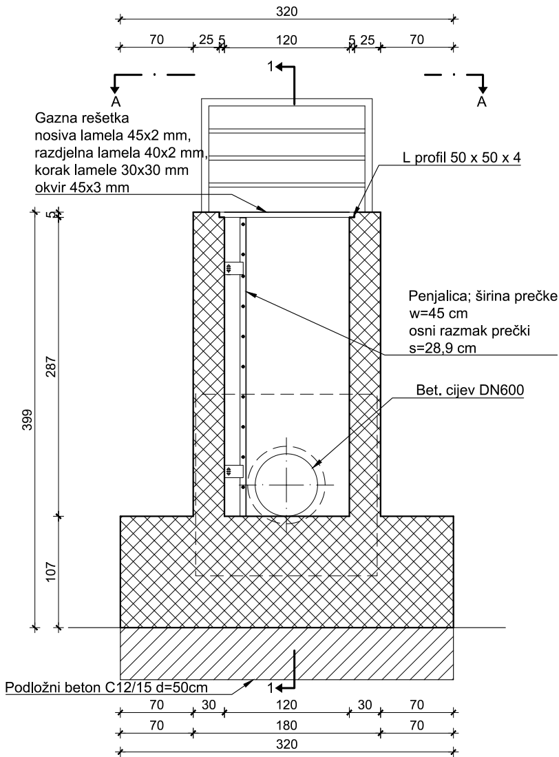
POPREČNI PRESJEK 4-4 M 1:50
