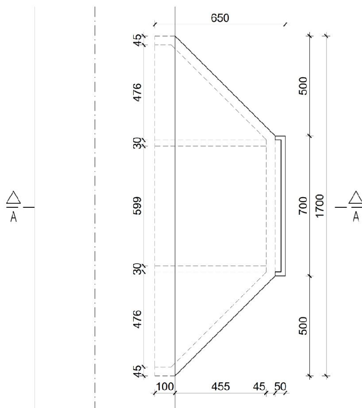
TLOCRT
