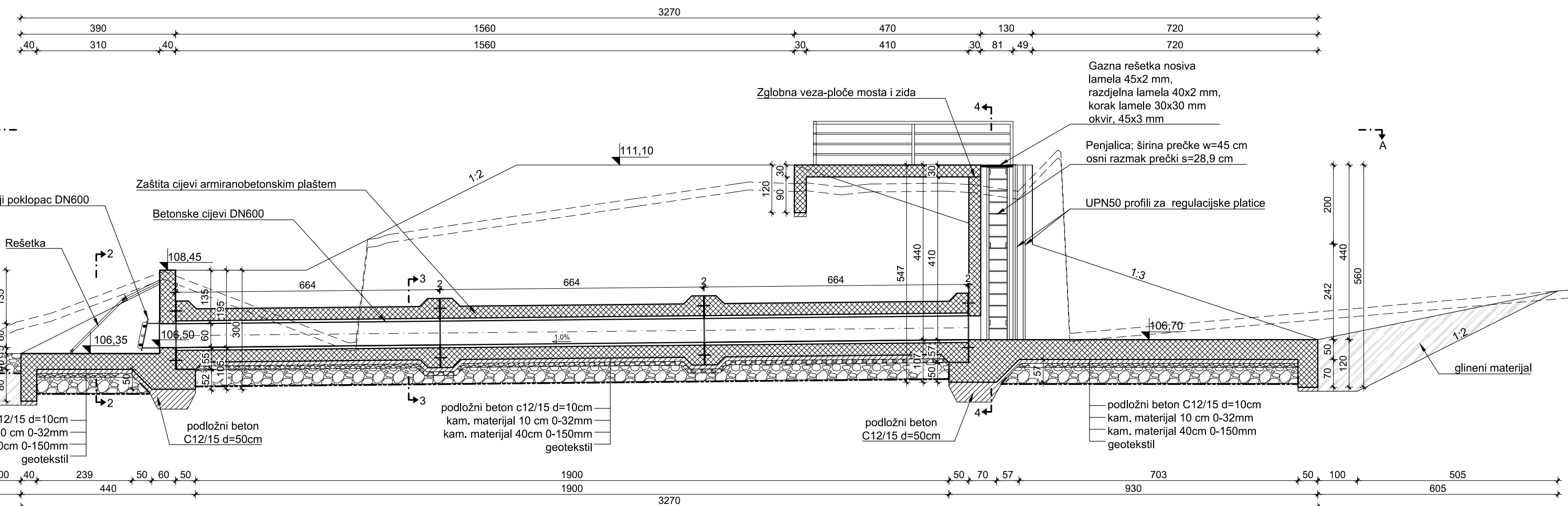
UZDUŽNI PRESJEK 1-1 M 1:100
