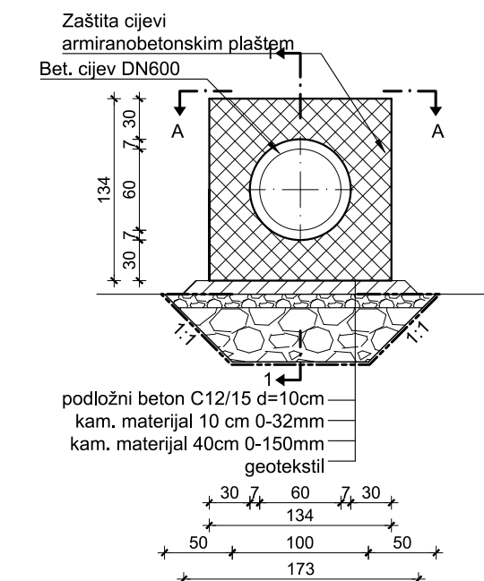
POPREČNI PRESJEK 3-3 M 1:50
