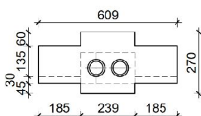
POPREČNI PRESJEK F-F
