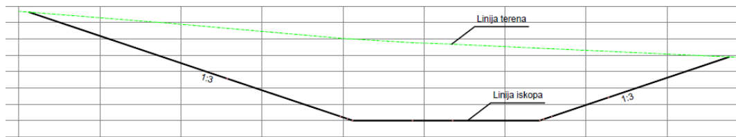
Slika 5-5: Uređenje nalazišta.
