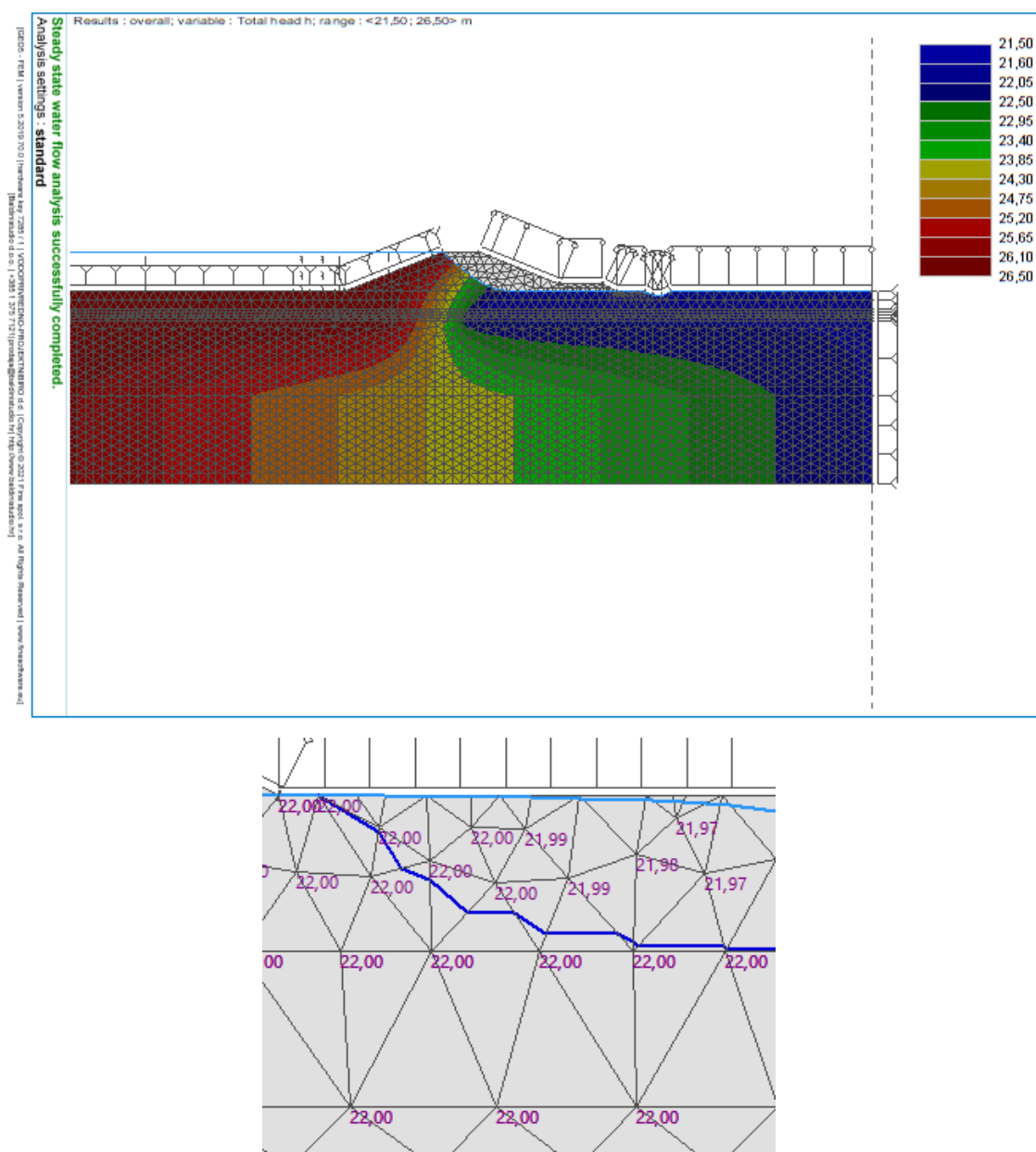
Slika 4-15: Rezultati analize procjeđivanja (iznos tlakova): H= 4,5 m, izvedba klina.
