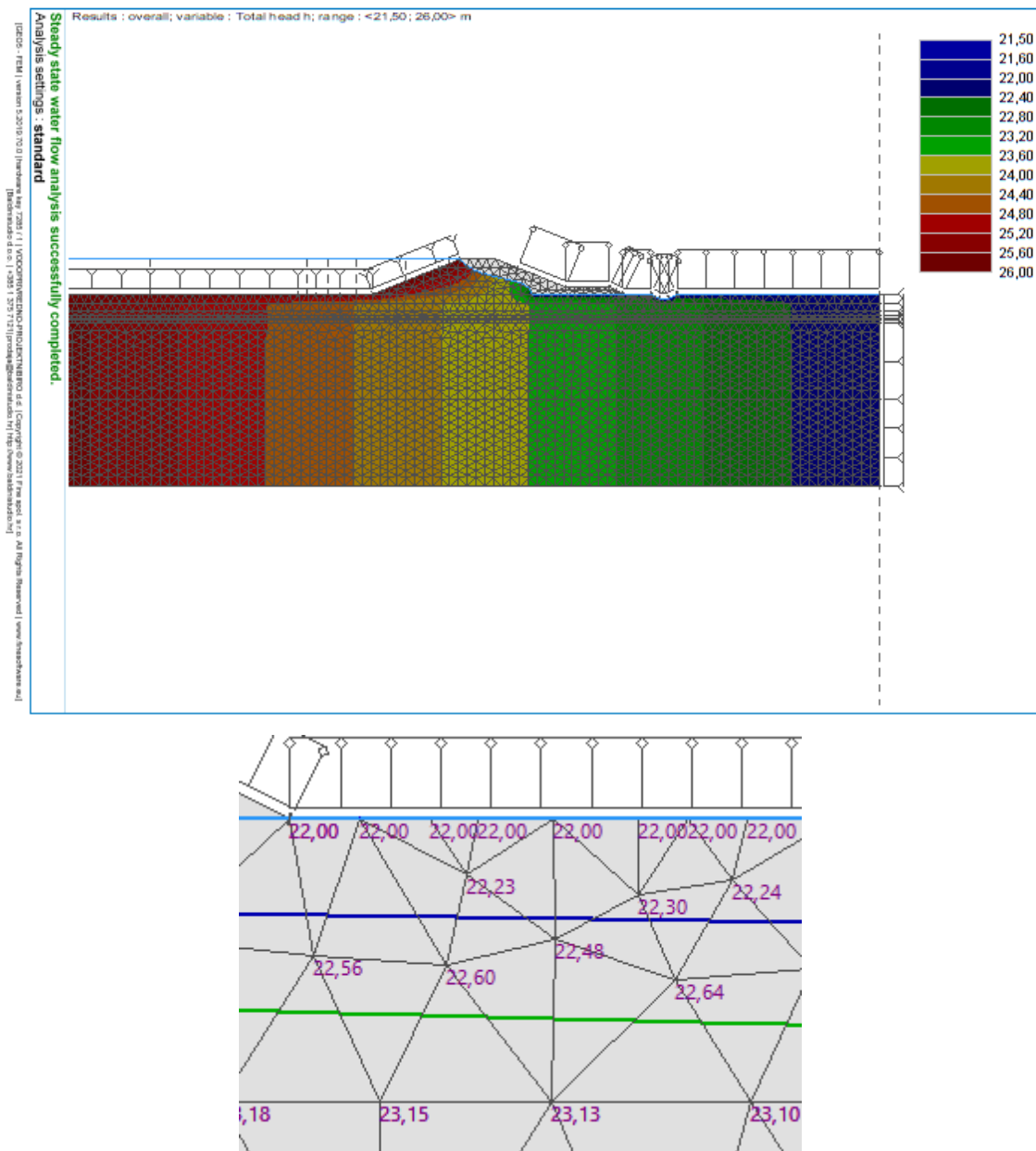
Slika 4-9: Rezultati analize procjeđivanja (iznos tlakova): H = 4,0 m, debljina sloja gline 1,0.
