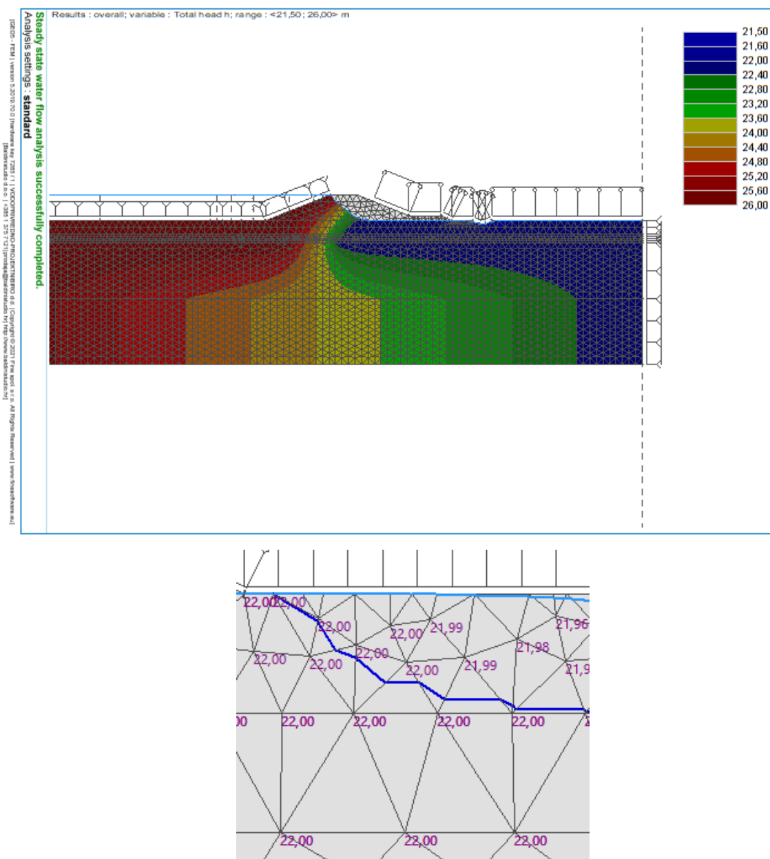
Slika 4-11: Rezultati analize procjeđivanja (iznos tlakova): H= 4,0 m, izvedba klina.
