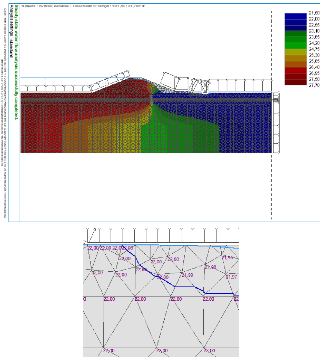
Slika 4-24: Rezultati analize procjeđivanja (iznos tlakova): H=5,7 m, izvedba nepropusne barijere.
