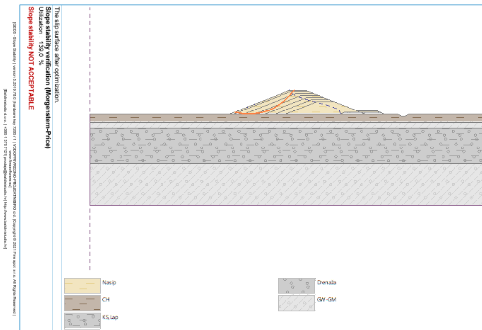
Slika 4-39: Nasip visine h = 5,7 m, klizna ploha za projektnu situaciju 3.
