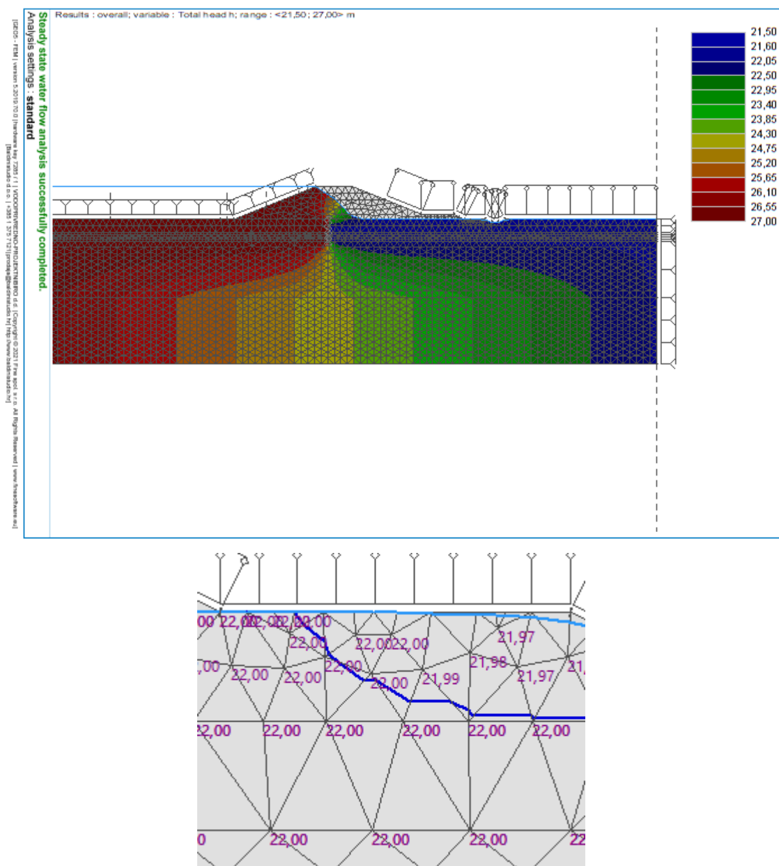
Slika 4-20: Rezultati analize procjeđivanja (iznos tlakova): H= 5,0 m, izvedba nepropusne barijere.
