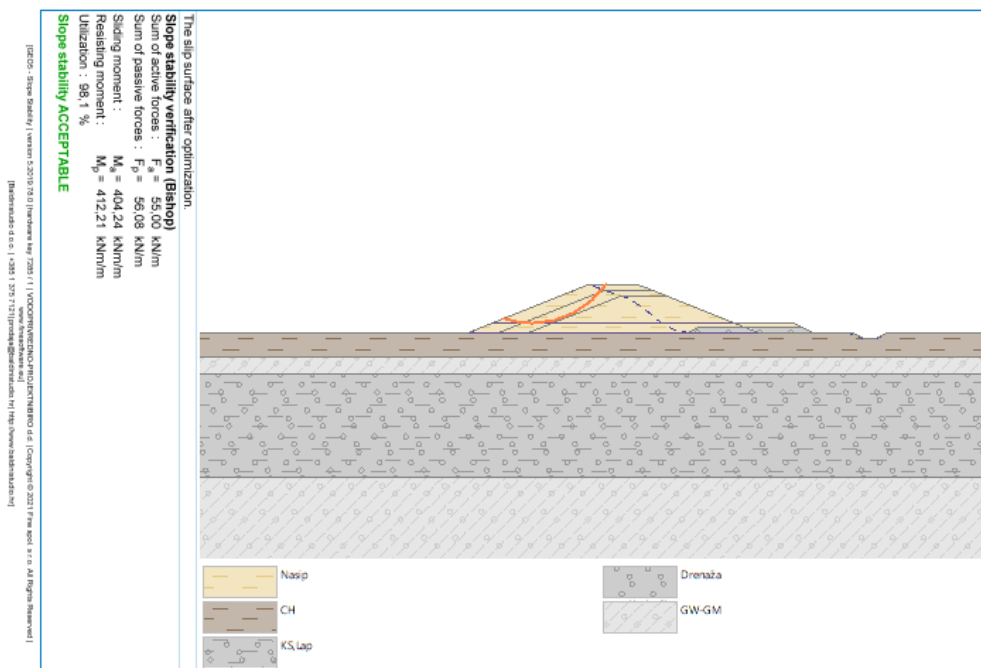
Slika 4-32: Nasip visine h = 4,0 m, klizna ploha za projektnu situaciju 4.
