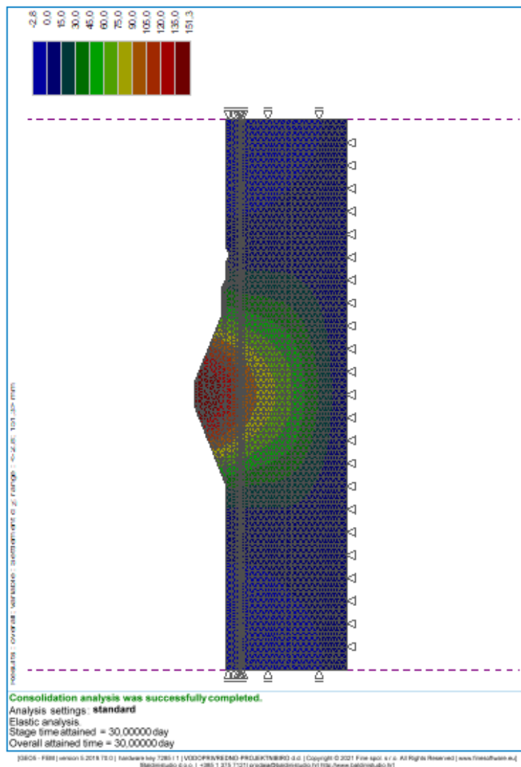
Slika 4-41: Nasip visine h = 5,7 m – slijeganje nakon 30 dana.
