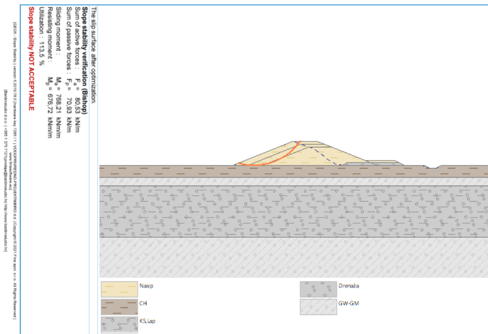
Slika 4-31: Nasip visine h = 4,0 m, klizna ploha za projektnu situaciju 3.
