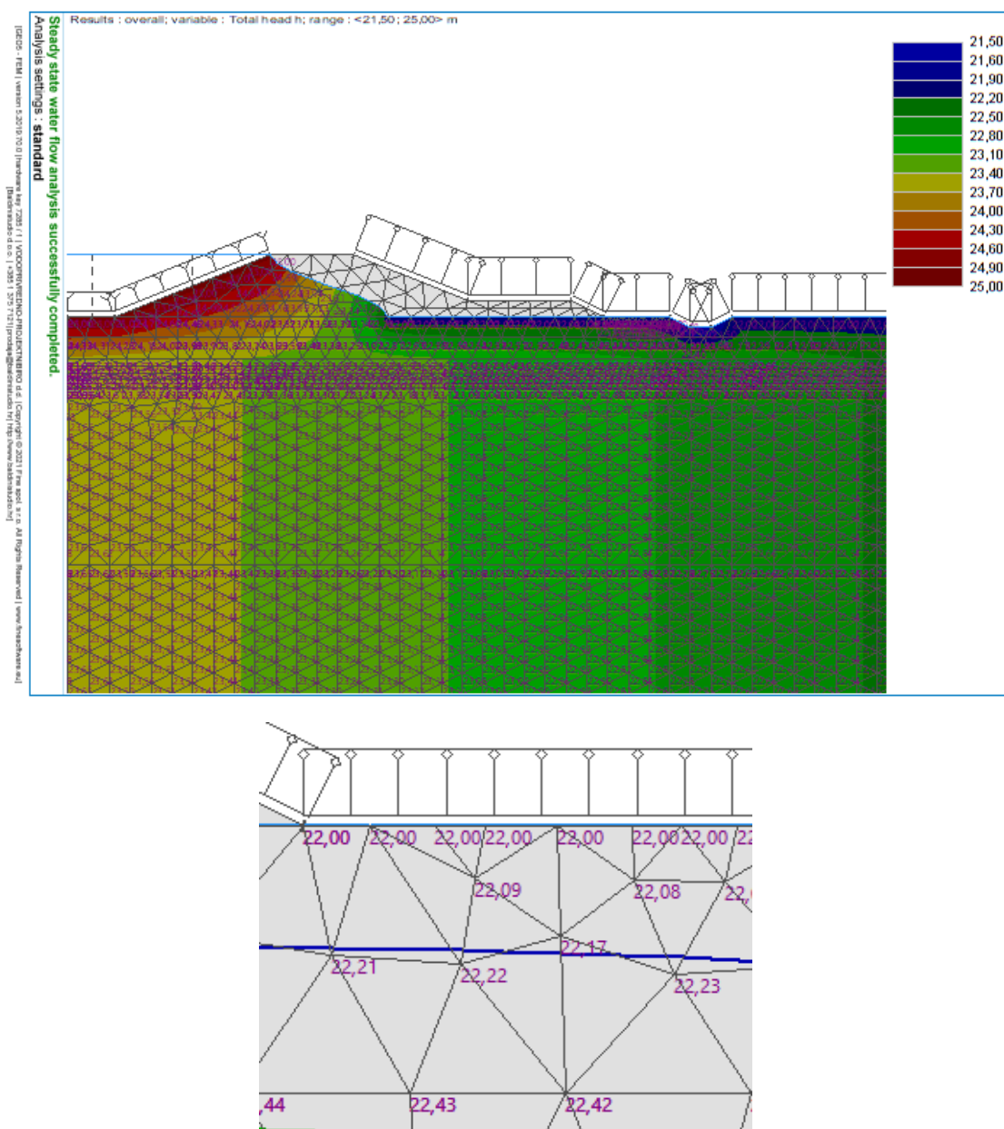
Slika 4-3: Rezultati analize procjeđivanja (iznos tlakova): H=3,0 m, debljina sloja gline 2,0.
