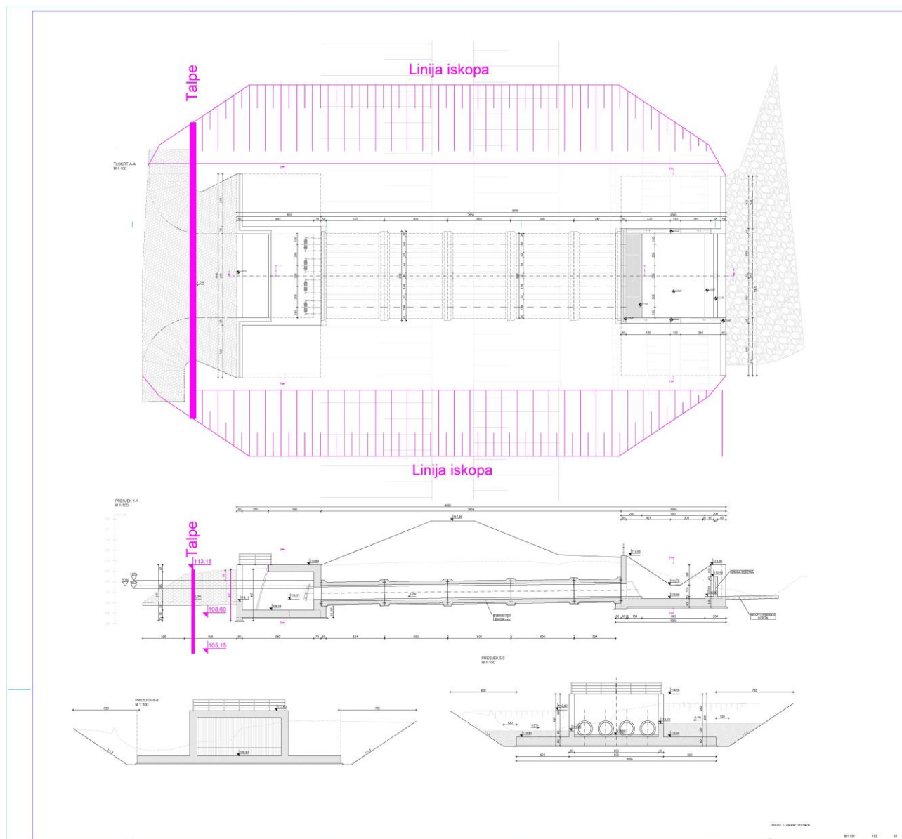
Slika 2-11: Talpe za zaštitu širokog iskopa od prelijevanja visokih voda.
