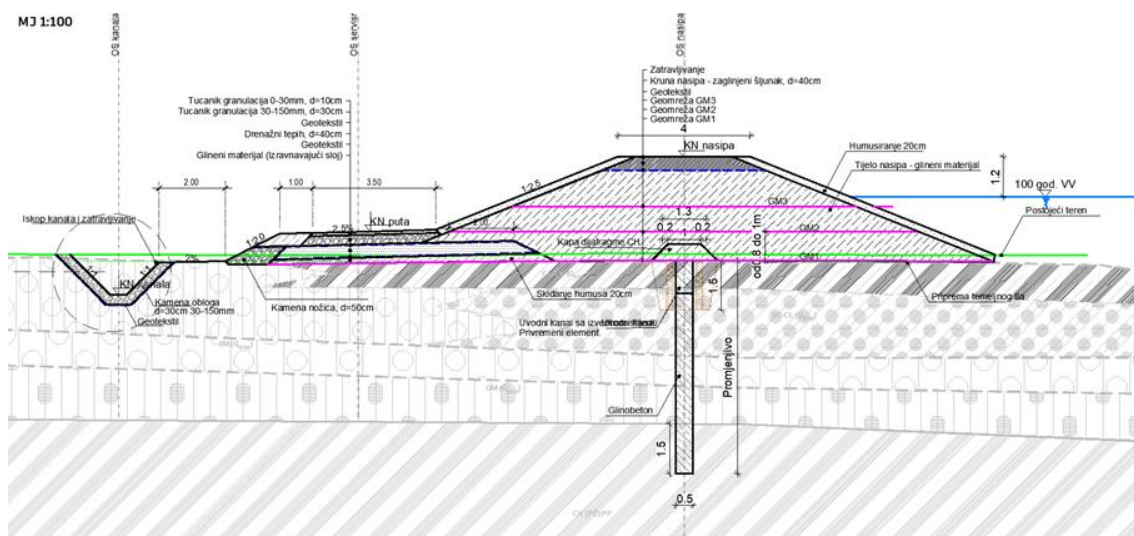
Slika 2-5: Karakteristični presjek 2 nasipa.
