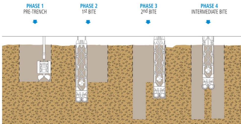
Slika 2-2: Raspored iskopa glavnih ( primarnih ) panela dijafragme.
