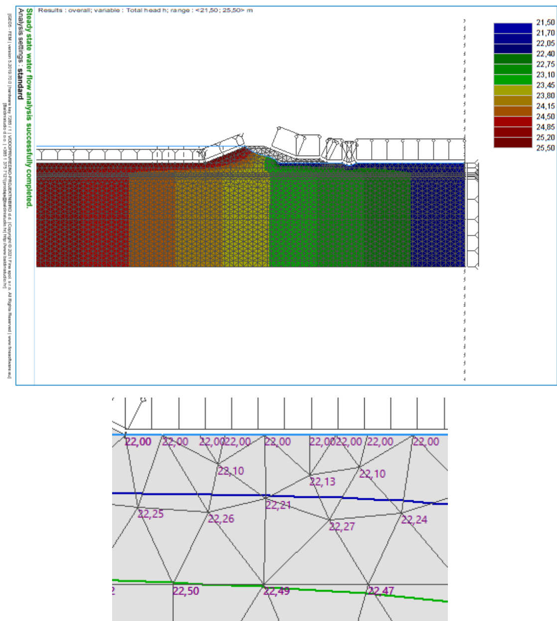
Slika 4-6: Rezultati analize procjeđivanja (iznos tlakova): H = 3,5 m, debljina sloja gline 2,0.
