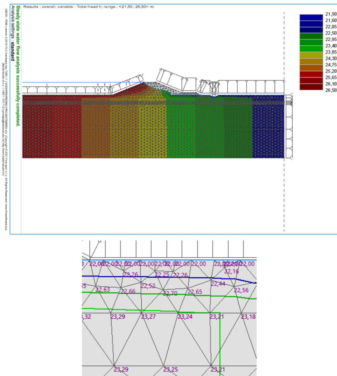
Slika 4-13: Rezultati analize procjeđivanja (iznos tlakova): H = 4,5 m, debljina gline 1,0.
