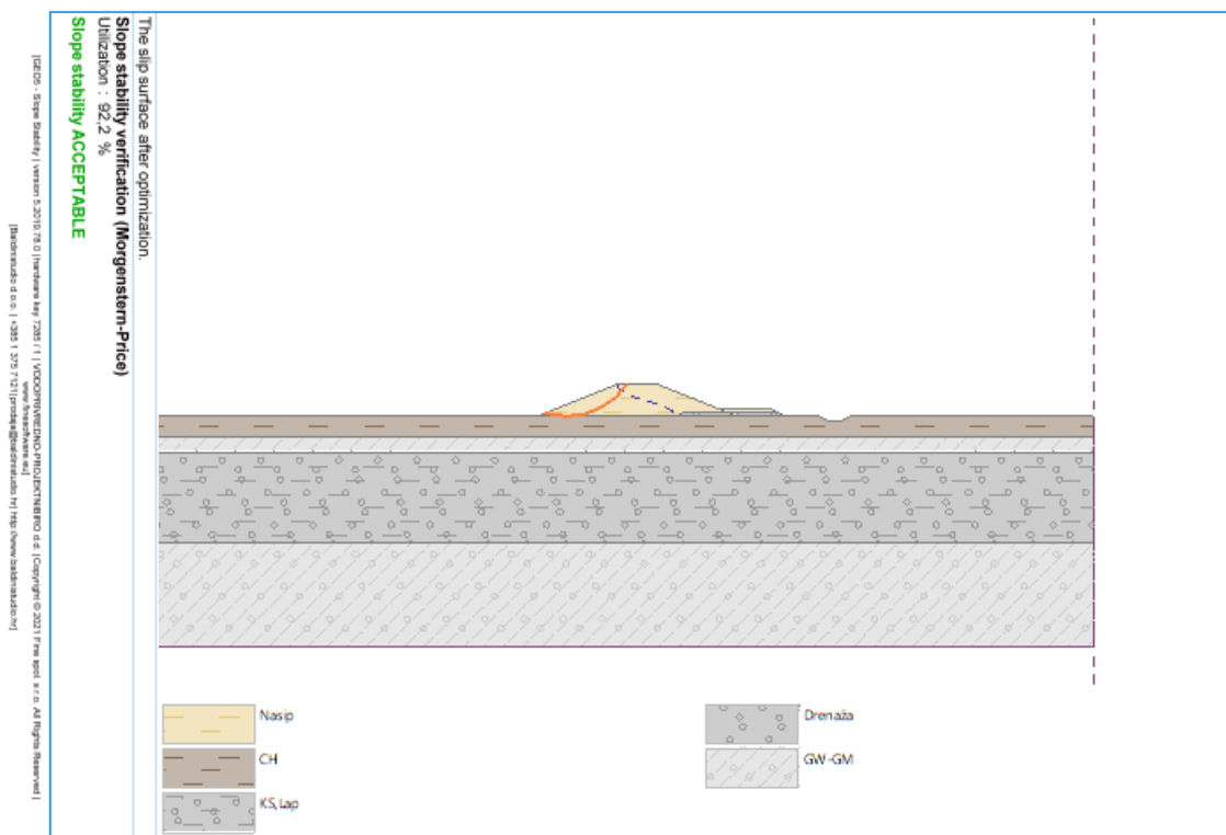
Slika 4-28: Nasip visine h = 3,0 m, klizna ploha za projektnu situaciju 3.
