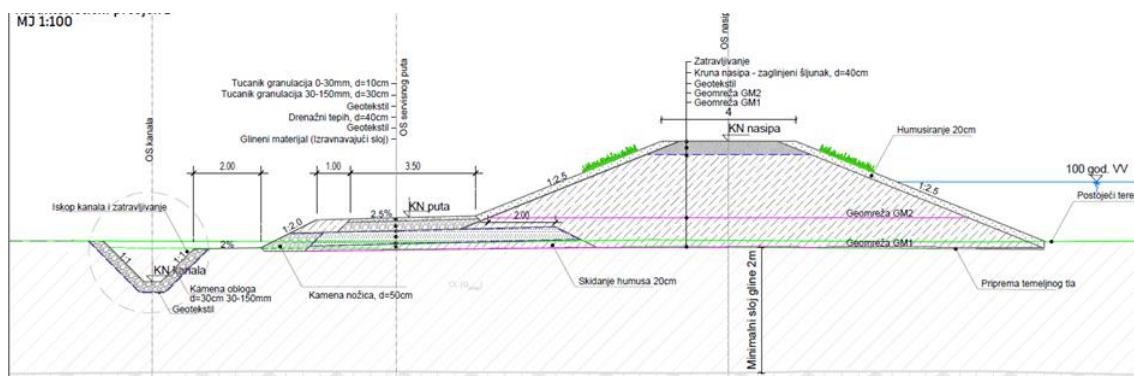
Slika 2-4: Karakteristični presjek 1 nasipa.
