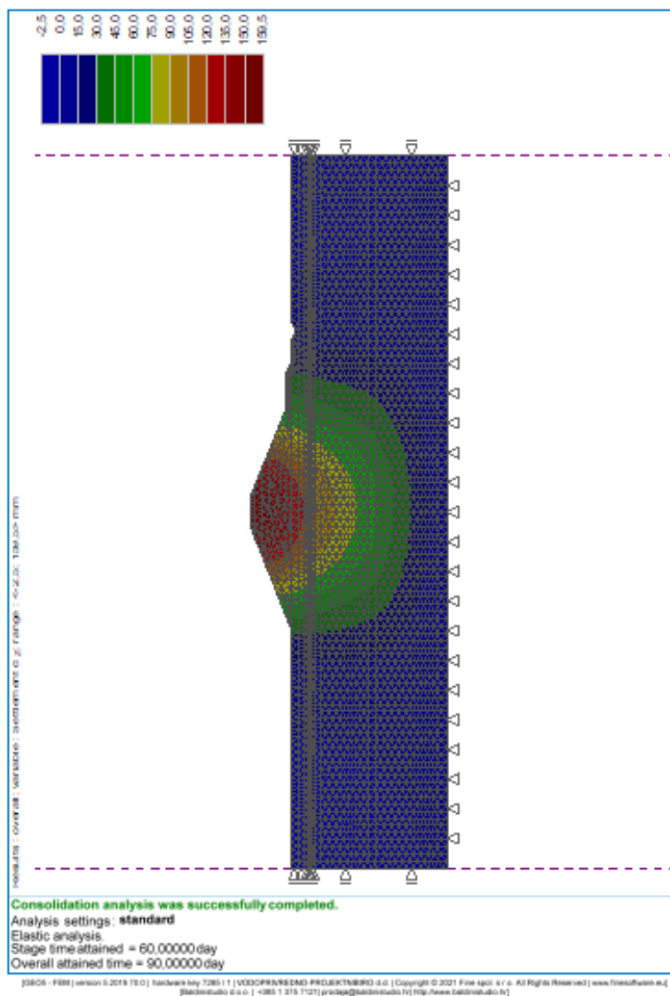
Slika 4-42: Nasip visine h = 5,7 m – slijeganje nakon 90 dana.
