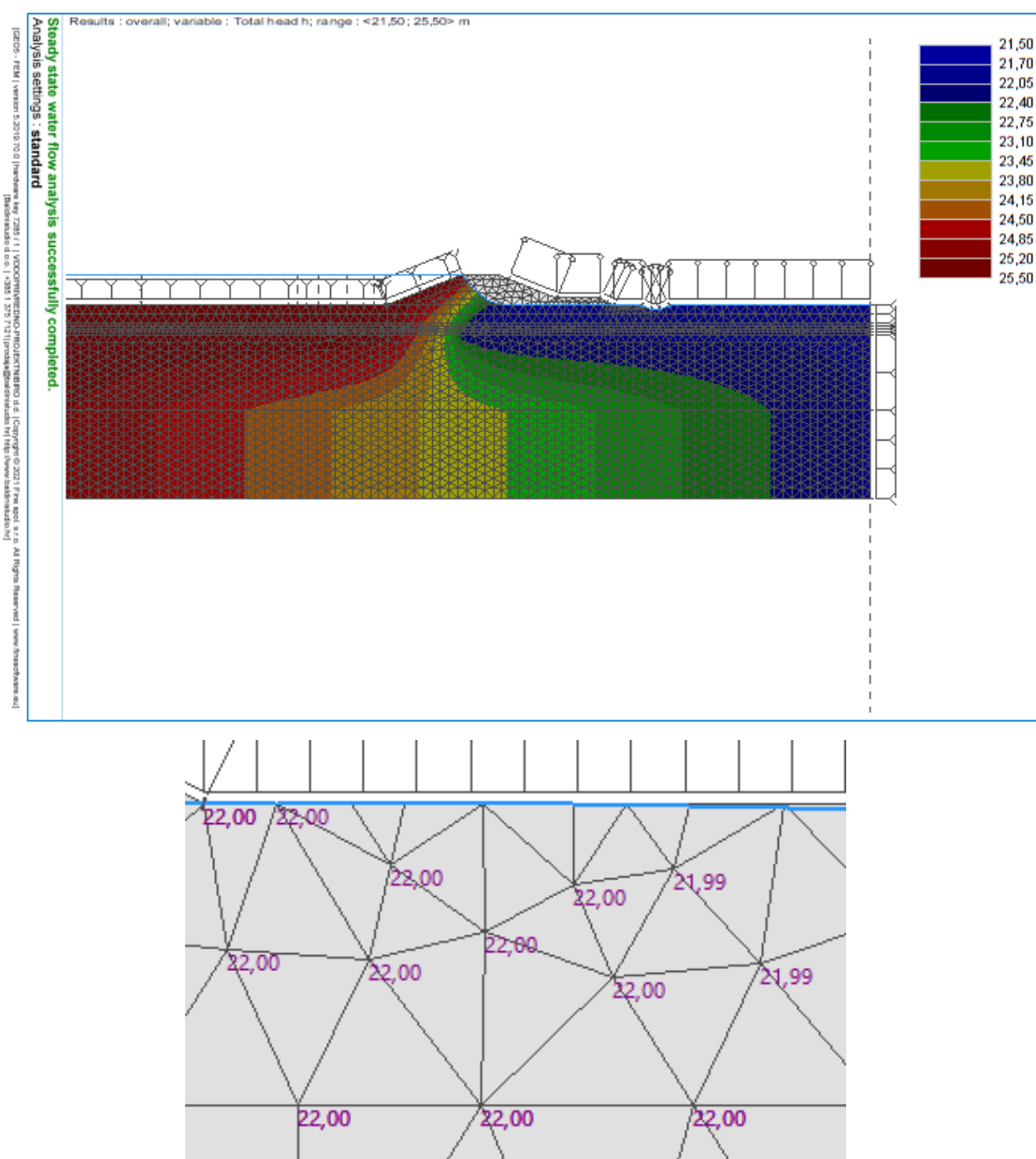
Slika 4-7: Rezultati analize procjeđivanja (iznos tlakova): H = 3,5 m, izvedeba klina.
