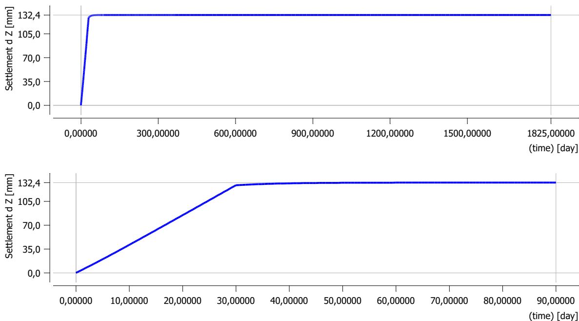
Slika 4-45: Nasip visine h = 5,7 m – slijeganje temeljnog tla tokom vremena.
