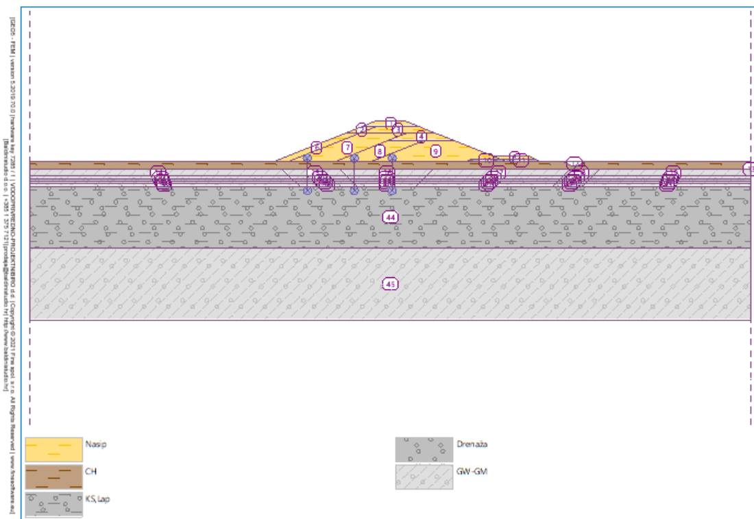
Slika 4-1: Model - Lijevi nasip Dobre.
