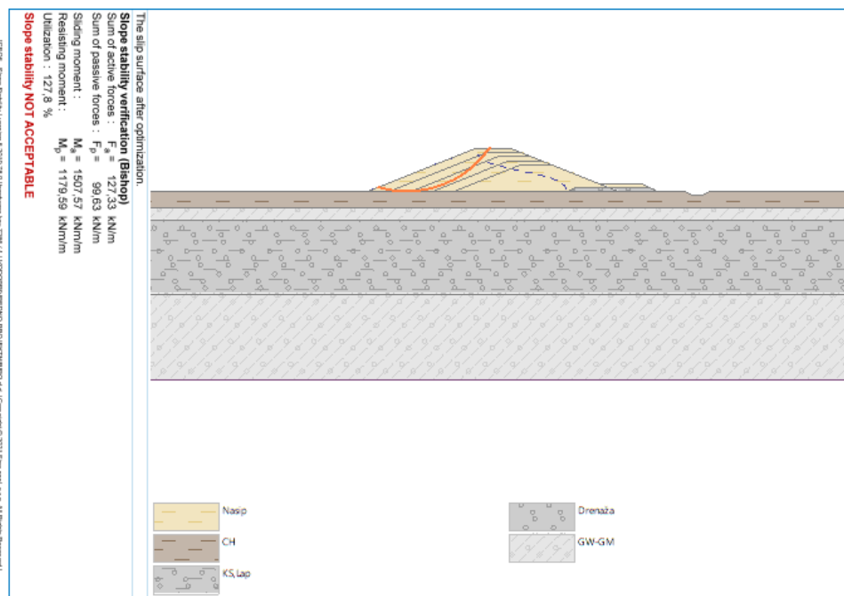
Slika 4-35: Nasip visine h = 5,0 m, klizna ploha za projektnu situaciju 3.
