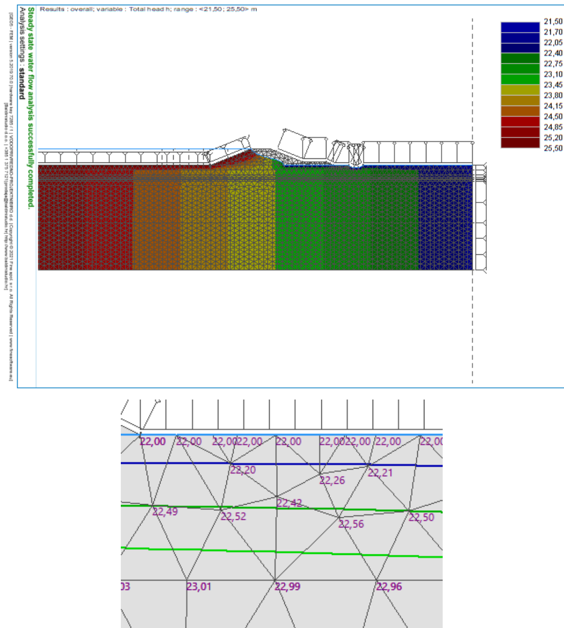
Slika 4-5: Rezultati analize procjeđivanja (iznos tlakova): H = 3,5 m, debljina sloja gline 1,0.
