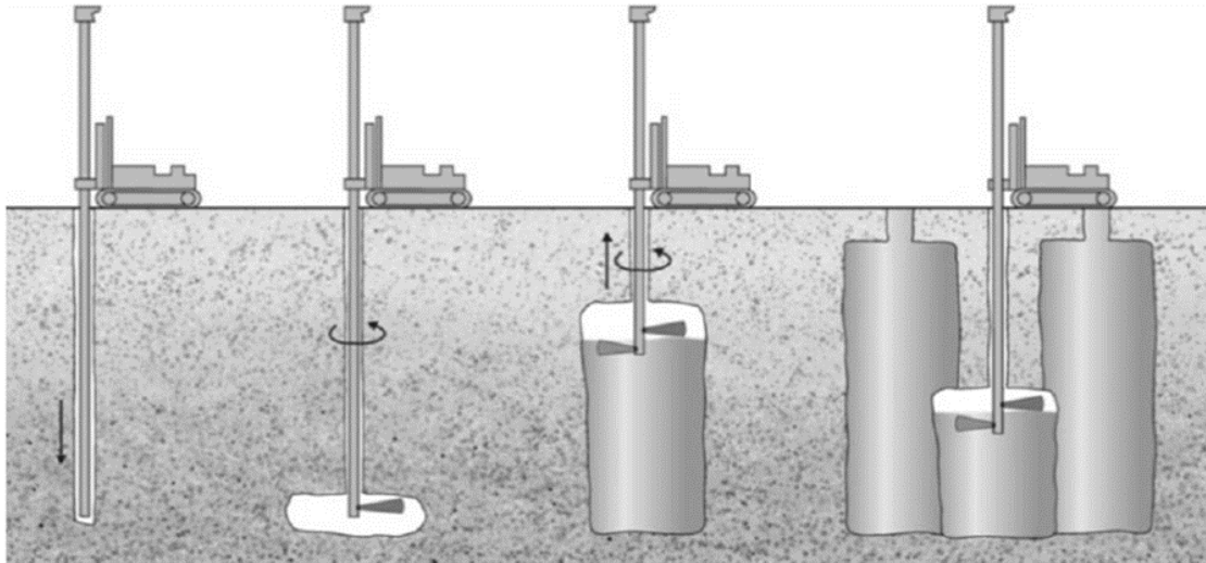
Slika 5-4: Redoslijed izvođenja mlaznog injektiranja (bušenje, rezanje, injektiranje i proširenje).
