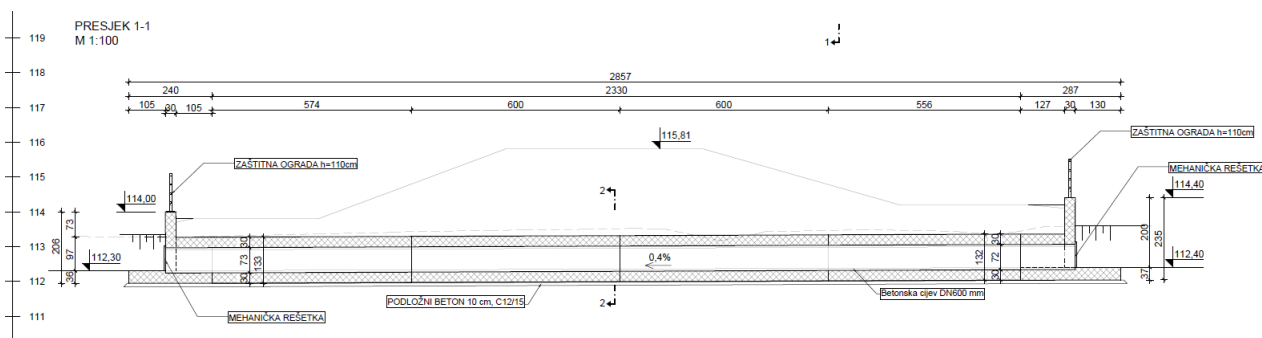
Slika 2-8: Karakteristični presjek propusta
