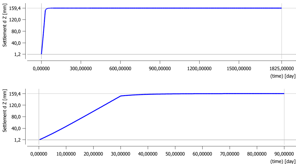
Slika 4-46: Nasip visine h = 5,7 m – slijeganje krune nasipa tokom vremena.
