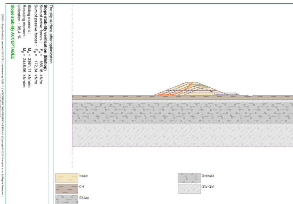
Slika 4-38: Nasip visine h = 5,5 m, klizna ploha za projektnu situaciju 4.
