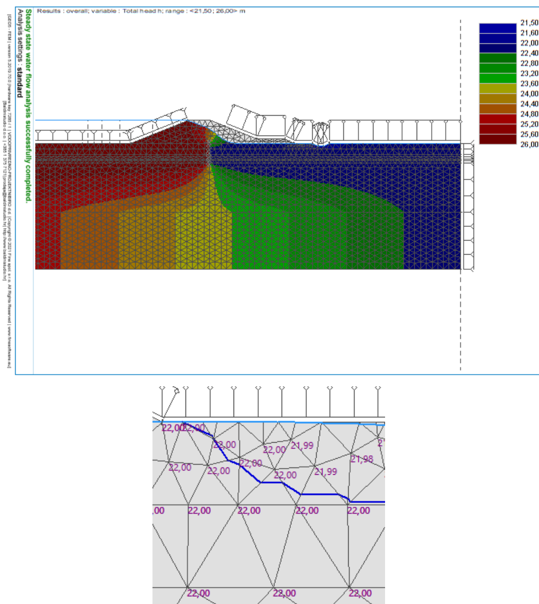
Slika 4-12: Rezultati analize procjeđivanja (iznos tlakova): H= 4,0 m, izvedba nepropusne barijere.
