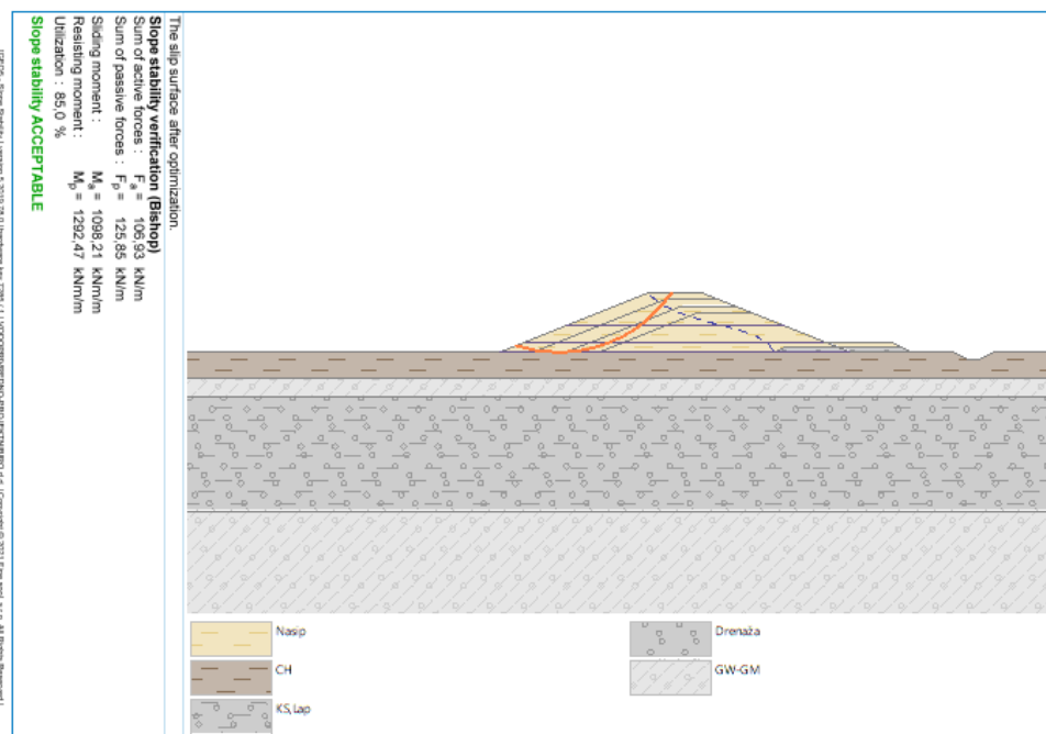
Slika 4-34: Nasip visine h = 4,5 m, klizna ploha za projektnu situaciju 4.
