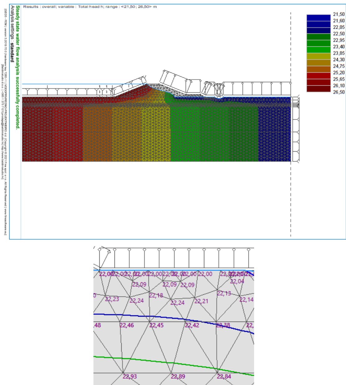
Slika 4-14: Rezultati analize procjeđivanja (iznos tlakova): H= 4,5 m, debljina gline 2,75.
