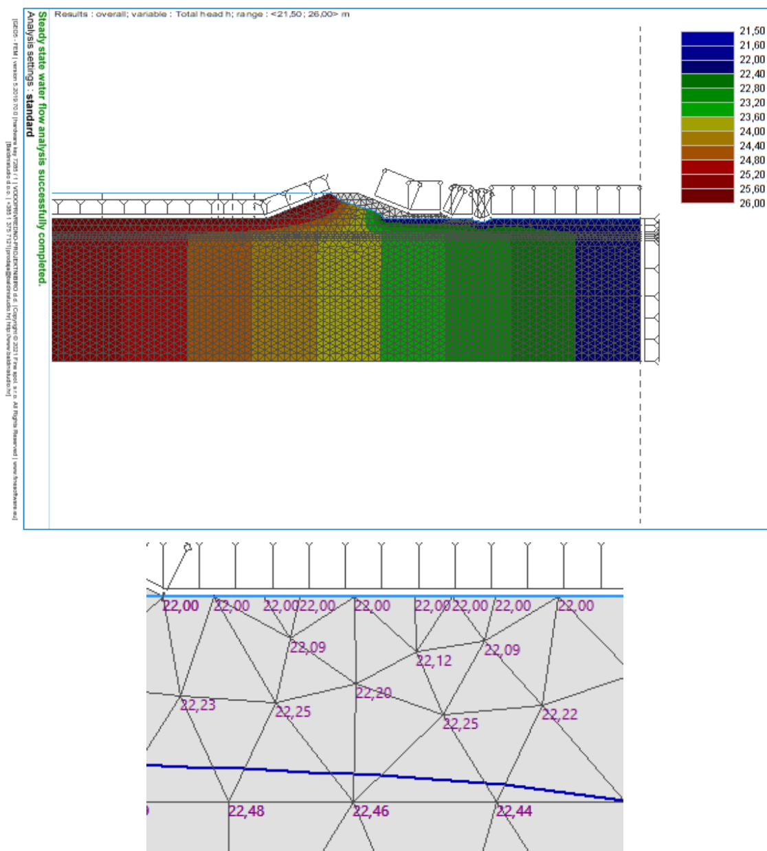
Slika 4-10: Rezultati analize procjeđivanja (iznos tlakova): H = 4,0 m, debljina sloja gline 2,4.
