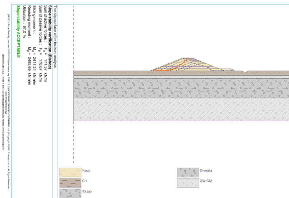
Slika 4-40: Nasip visine h = 5,7 m, klizna ploha za projektnu situaciju 4.
