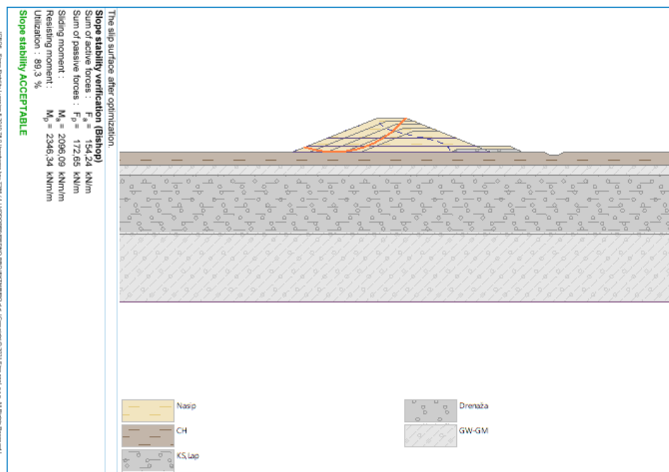
Slika 4-36: Nasip visine h = 5,0 m, klizna ploha za projektnu situaciju 4.
