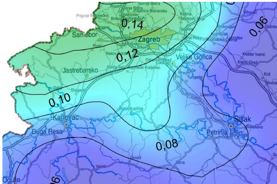
Slika 4-25: Poredbeno vršno ubrzanje tla tipa A ( a_{gR} ), s vjerojatnosti premašaja 10 % u 10 godina, za poredbeno povratno razdoblje potresa T_{DLR} = 95 godina, izraženo u jedinicama gravitacijskog ubrzanja ( g )
