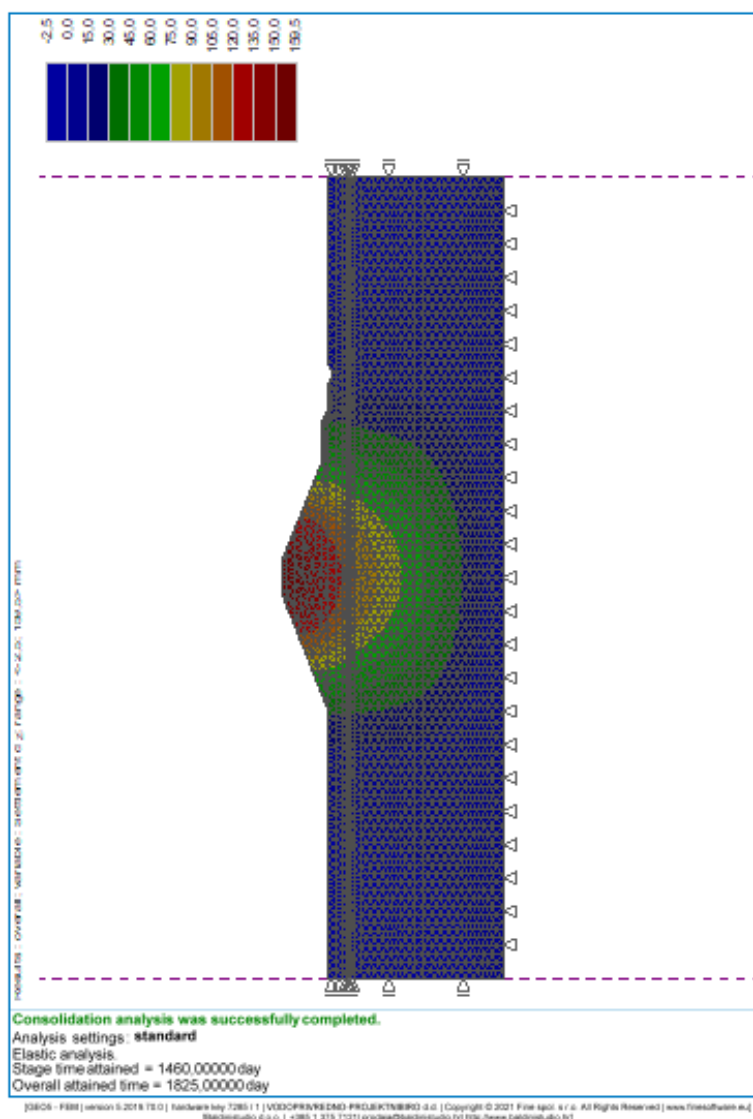
Slika 4-44: Nasip visine h = 5,7 m – slijeganje nakon 1825 dana.
