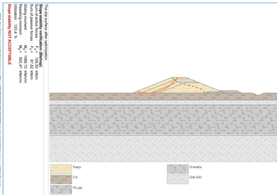
Slika 4-33: Nasip visine h = 4,5 m, klizna ploha za projektnu situaciju 3.
