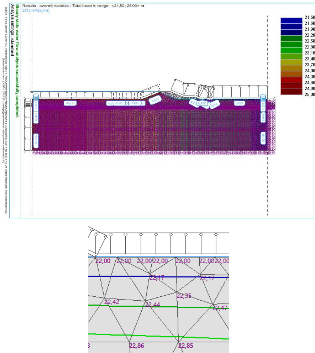
Slika 4-2: Rezultati analize procjeđivanja (iznos tlakova): H = 3,0 m, debljina sloja gline 1,0.
