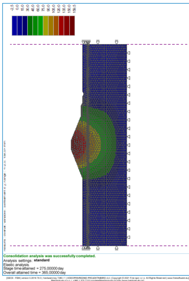
Slika 4-43: Nasip visine h = 5,7 \text{ m} – slijeganje nakon 365 dana.
