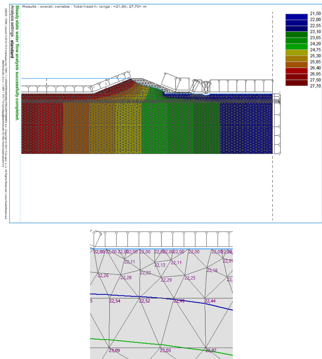
Slika 4-22: Rezultati analize procjeđivanja (iznos tlakova): H=5,7 m, debljina gline 3,0.
