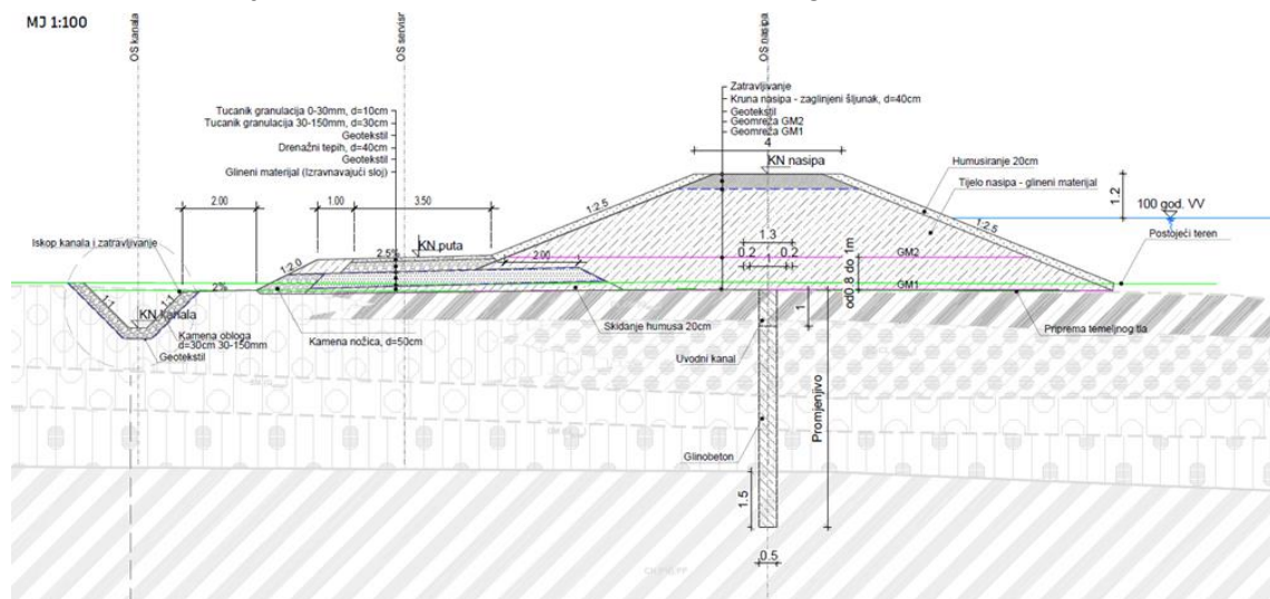
Slika 2-1: : Karakteristični profil nasipa.
