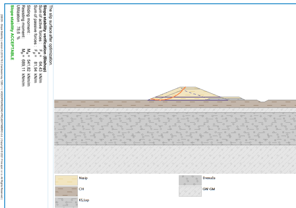
Slika 4-30: Nasip visine h = 3,5 m, klizna ploha za projektnu situaciju 4.
