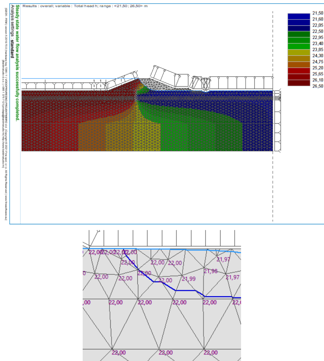
Slika 4-16: Rezultati analize procjeđivanja (iznos tlakova): H = 4,5 m, izvedba nepropusne barijere.
