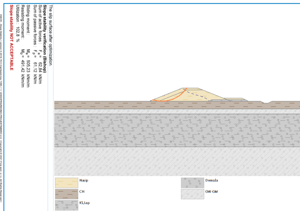
Slika 4-29: Nasip visine h = 3,5 m, klizna ploha za projektnu situaciju 3.
