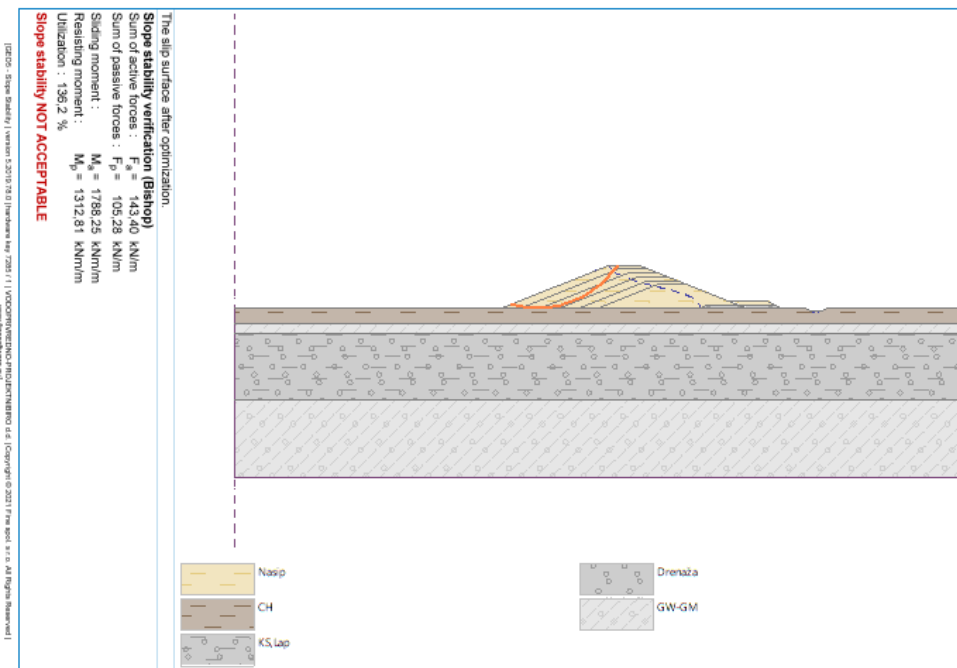
Slika 4-37: Nasip visine h = 5,5 m, klizna ploha za projektnu situaciju 3.
