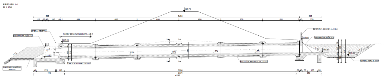
Slika 2-7: Karakteristični presjek ispusta
