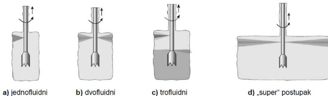
Slika 5-3: Sustavi mlaznog injektiranja.
