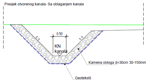
Slika 2-6: Karakteristični presjek otvorenog kanala.
