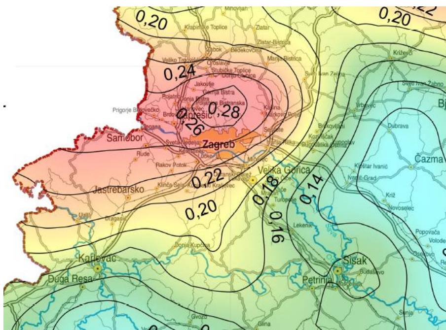
Slika 4-26: Poredbeno vršno ubrzanje tla tipa A ( a_{gR} ), s vjerojatnosti premašaja 10 % u 50 godina, za poredbeno povratno razdoblje potresa T_{NCR} = 475 godina, izraženo u jedinicama gravitacijskog ubrzanja (g)
