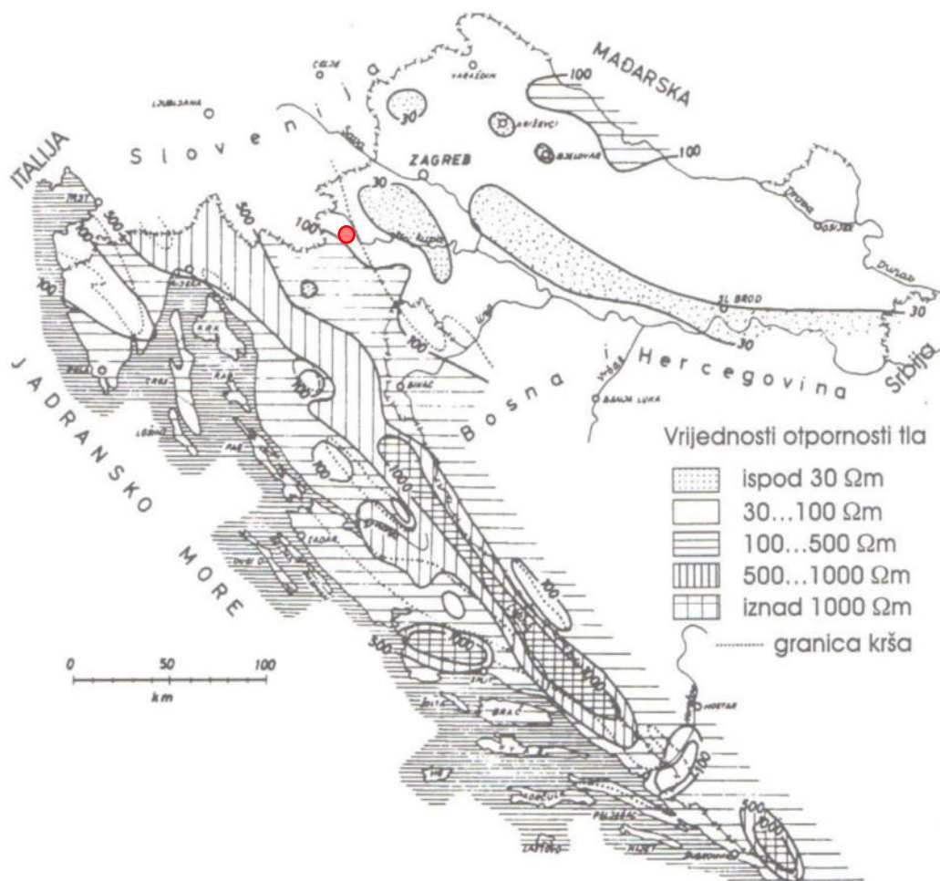
Slika 1: Orijentacijska karta otpornosti tla na dubini od 1 m za područje Hrvatske (izvor: Uzemljivači i sustavi uzemljena, Majdandžić Franjo, Zagreb: Graphis, 2004.)
