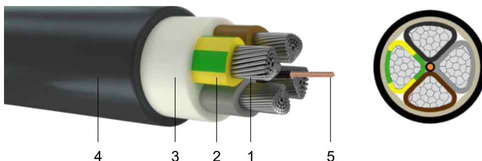
Slika 2: Konstrukcija NN kabela NA2XY-O
