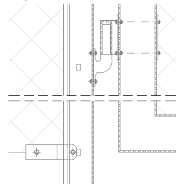
Detalj "D1" - šarke i zatezač žice M: 1:5
